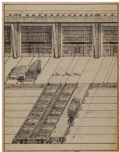
Dessin du chariot de translation avec ses quatre rails spéciaux et du tracteur-poussoir, croquis XII (Service Historique de la Défense de Lorient, Monographie de la base "Ingénieur Général Stoskopf", 1945-1946) Phot. Service Historique de la Défense IVR53_20225606364NUCA
