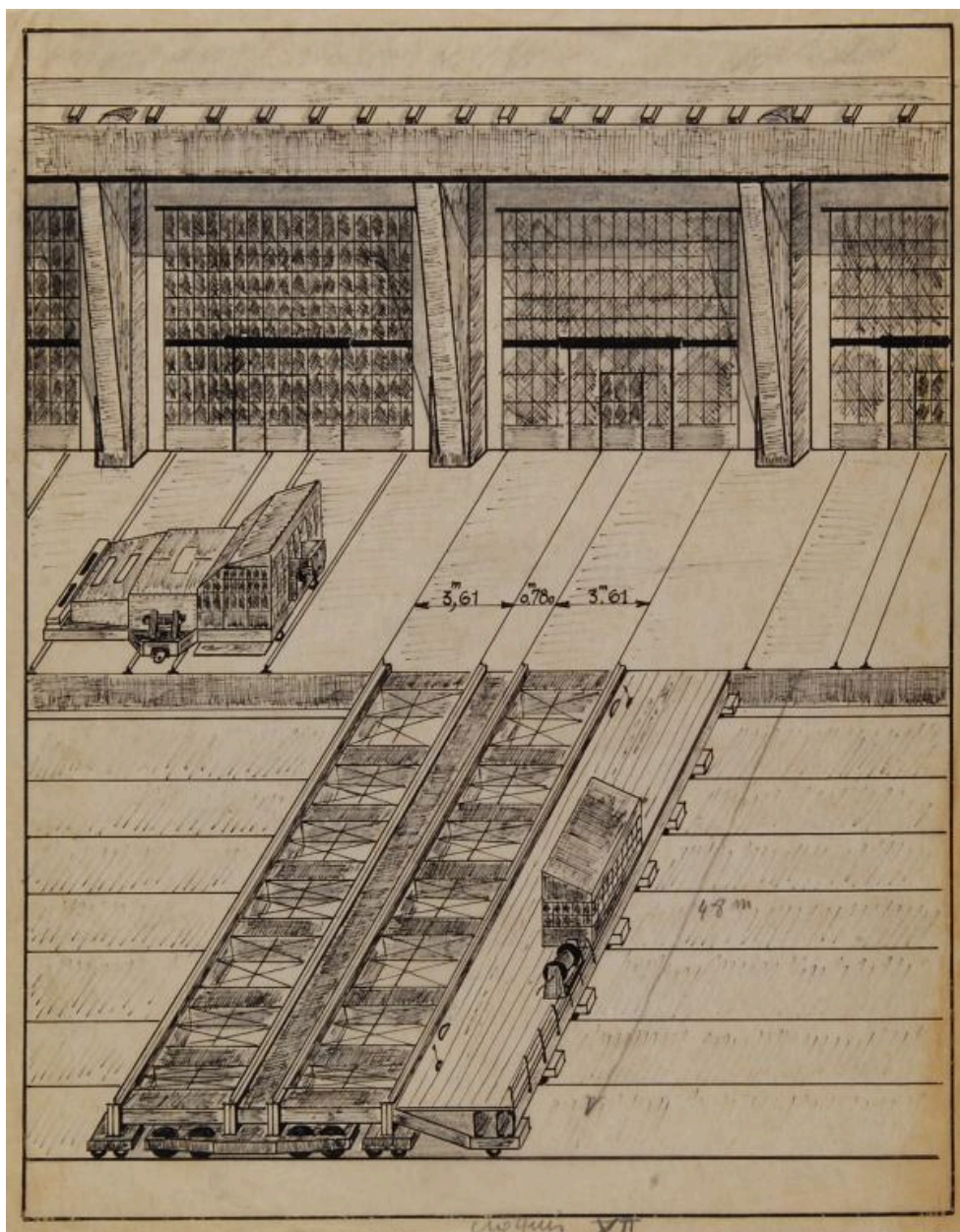
Dessin du chariot de translation avec ses quatre rails spéciaux et du tracteur-pousseur, croquis XII (Service Historique de la Défense de Lorient, Monographie de la base "Ingénieur Général Stosskopf", 1945-1946)
