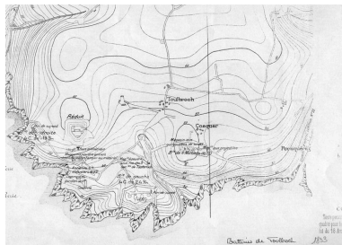
Plan de l'ensemble fortifié de Toulbroc'h, Atlas des batteries de côte, n° 20 : côte de Brest, 1893, Vincennes Repro. Guillaume Lécueillier IVR53_20032901706NUCA
