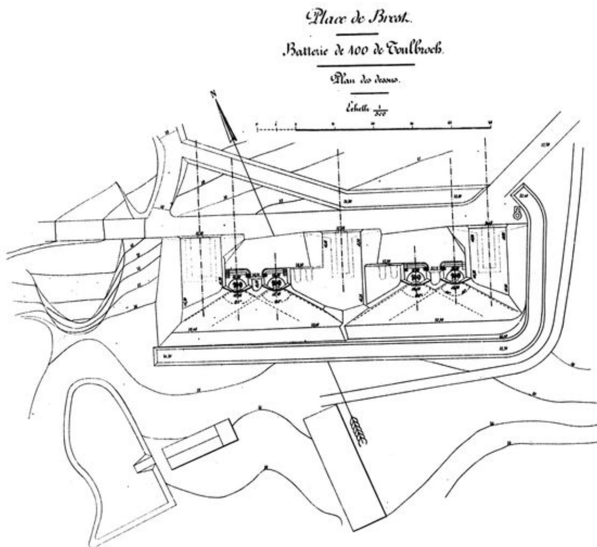
Plan de la batterie de 100 mm de Toulbroc'h
