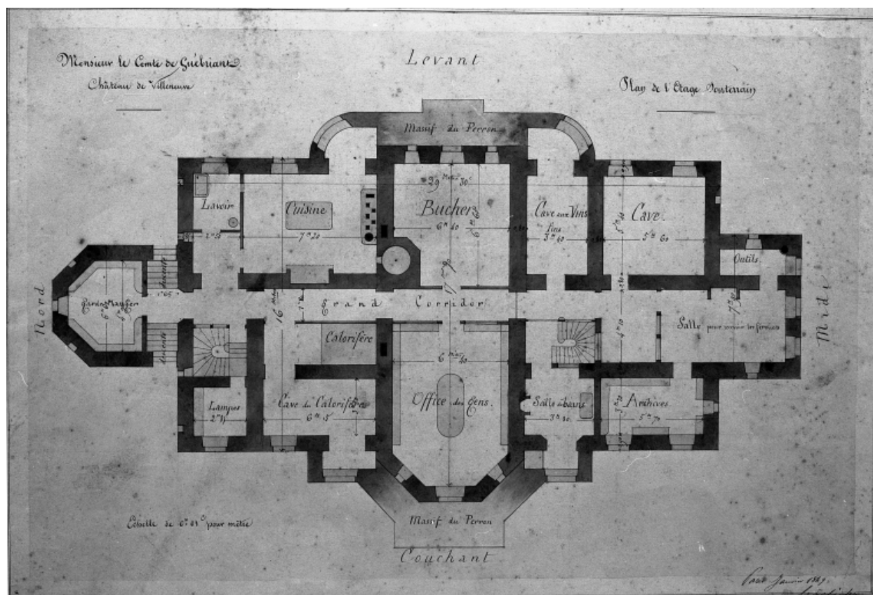
Plan du sous-sol : projet par Froelicher en 1848 (coll. privée)
