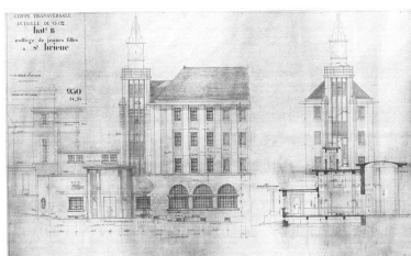
Élévations et coupe du bâtiment B (internat et tour), G-R. Lefort, architecte, 15 janvier 1936. Noter, entre autres, l'emplacement réservé aux décorations. Dess. Georges-Robert Lefort IVR53_20182206109A0
