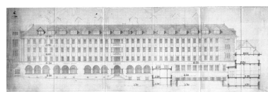
Élévations des façades de la tour, de l'internat et coupe du réfectoire, G-R. Lefort, architecte, sd. Dess. Georges-Robert Lefort IVR53_20182206107A0
