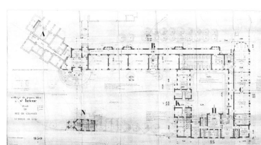
Bâtiments construits à partir de 1936 (G-R. Lefort, architecte) : plans du rez-de-chaussée de la "tour", de l'internat, du réfectoire, des cuisines, de l'économat (modifié avant réalisation) et de la loge d'entrée. Dess. Georges-Robert Lefort IVR53_20182206106A0
