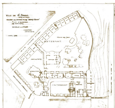
Plan masse, avril 1938. Dess. Georges-Robert Lefort IVR53_20182206104A0
