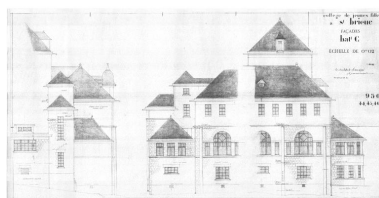
Elévations des façades du réfectoire, G-R. Lefort, architecte, janvier 1936. Dess. Georges-Robert Lefort IVR53_20182206108A0
