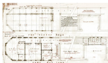
Plan des sous-sol et rez-de-chaussée de l'extension. G-R. Lefort, architecte, 11 septembre 1951. Dess. Georges-Robert Lefort IVR53_20182206115A0
