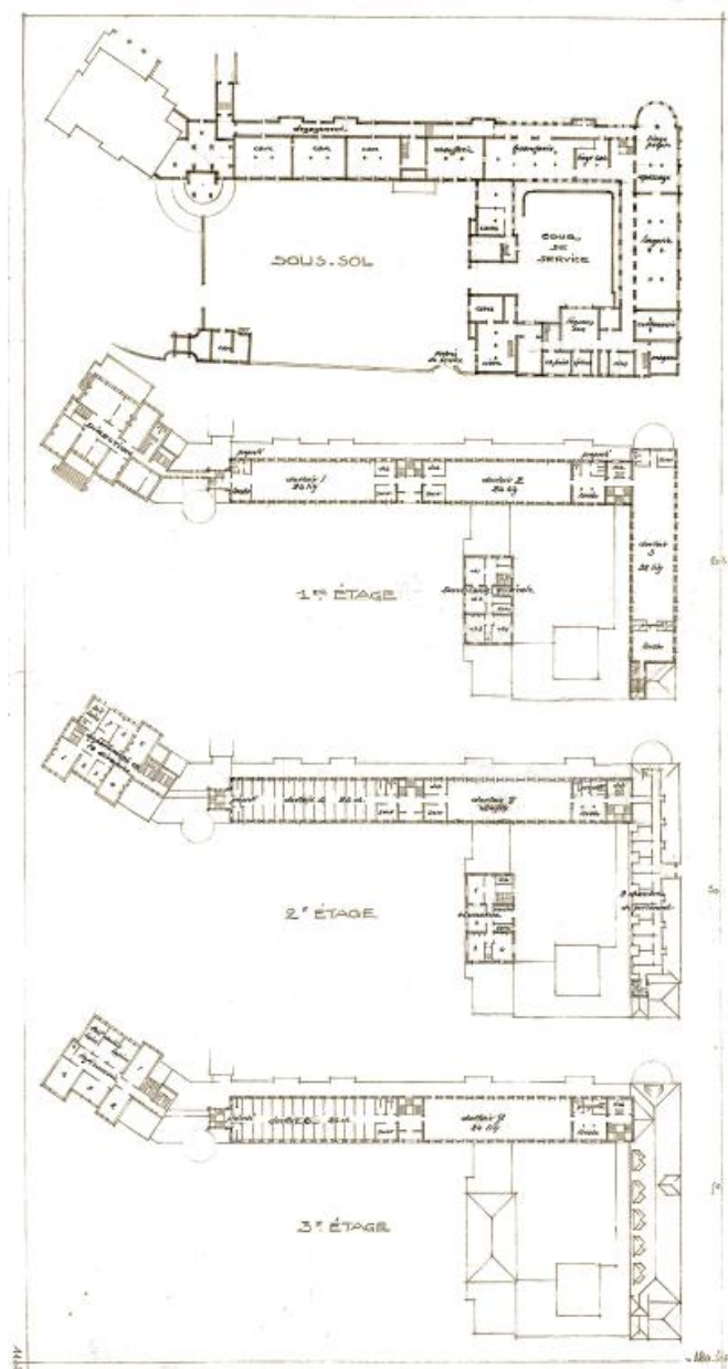
Plan des différents niveaux de la villa Baratoux, de l'internat, de l'économat, du réfectoire, des cuisines et de la loge. G-R. Lefort, architecte (sd. ca 1936)
