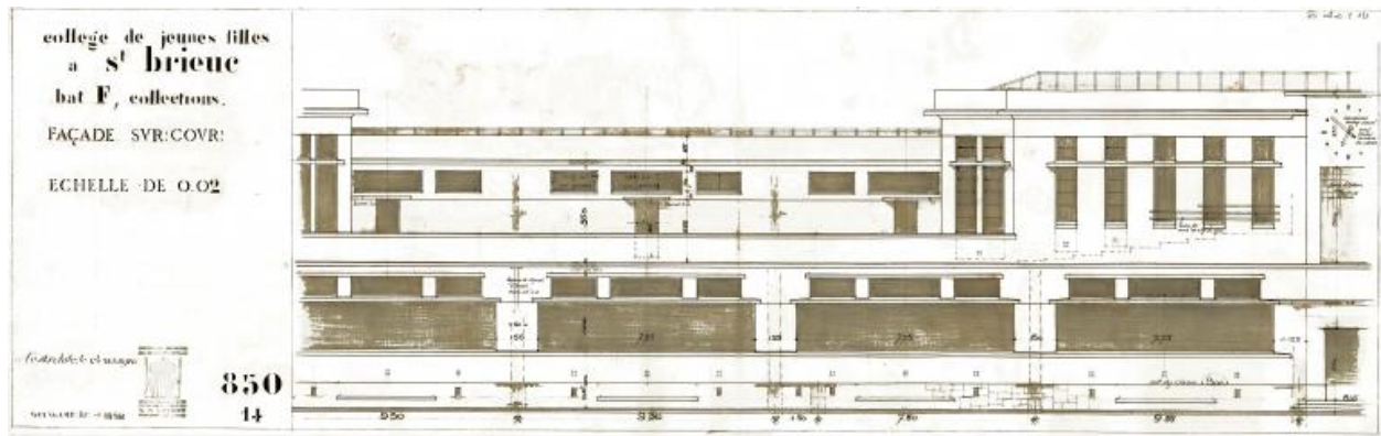
Élévation façade sur cour, G-R Lefort, 1934
