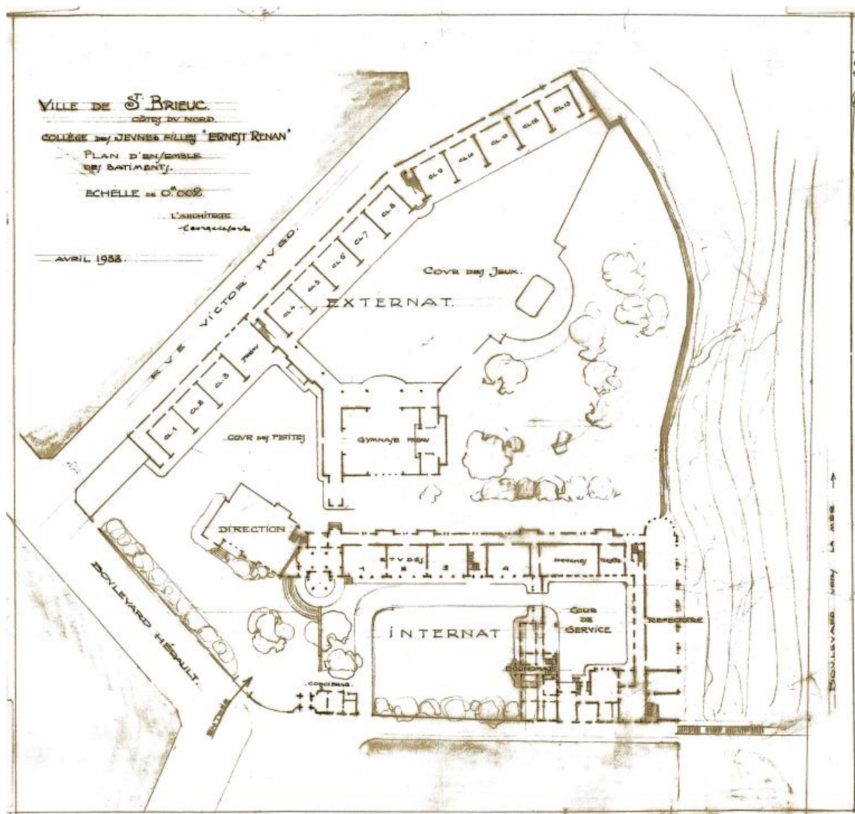
Plan masse, avril 1938.
