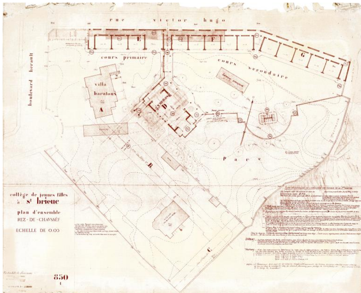
Plan masse, 1934.
