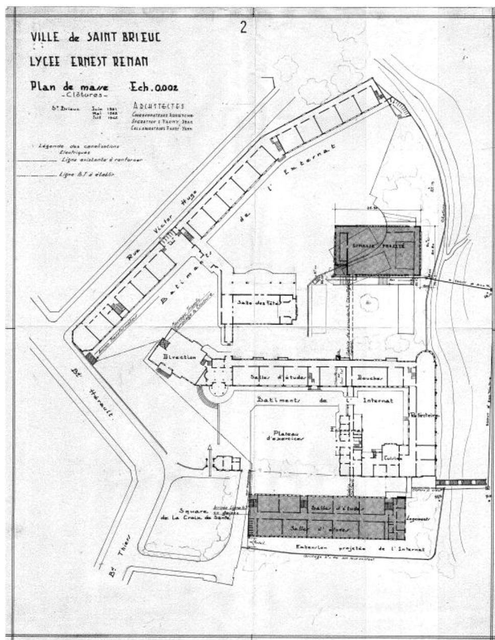
Plan de masse, juillet 1962, avec gymnase projeté et extension projetée de l'internat. Coordonnateur : Arretche, opération : Jean Fauny, collaborateur : Yann Fauny.
