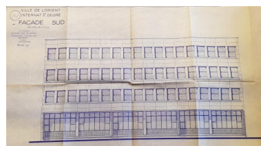
Internat : élévation de la façade sud (G. Tourry architecte chef)
