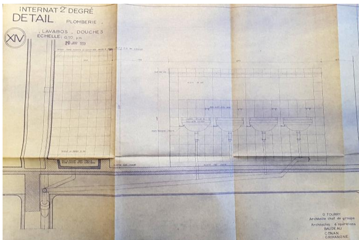
Internat : Détail, douches et lavabos (G. Tourry architecte chef de groupe, Baudeau, Conan, Brihangne, architectes, 20/01/1953).
