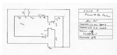
Plan du bunker-abri de type VF 1b pour 6 soldats (dessin : Dirk Peeters) Phot. Dirk Peeters IVR53_20252910607NUC
