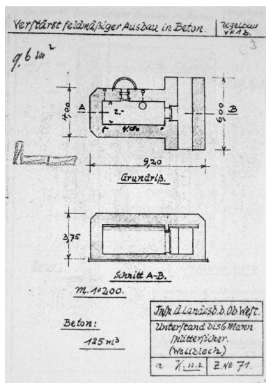
Plan d'un bunker - casemate de type VF 1b (Verstärkt feldmässiger Ausbau in Beton, Regelbau VF1b : Unterstand bis 6 Mann, Splittersicher [pare- éclats], Wellblech [tôle ondulée]) Repro. Guillaume Lécueillier IVR53_20252910599NUC
