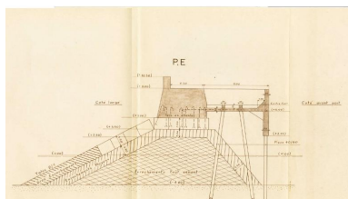
Prolongement sur 140m de longueur du môle de la pierre glissante à la pointe de Ste Barbe ; profils en travers (30/06/1964 ; projet) Phot. Ponts-et-Chaussées IVR53_20232905867NUCA
