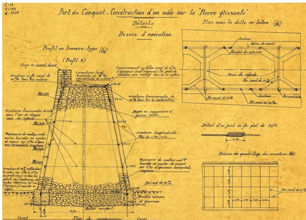
Plan et dessin d'exécution de la construction du môle sur la pierre-glissante (1928)
