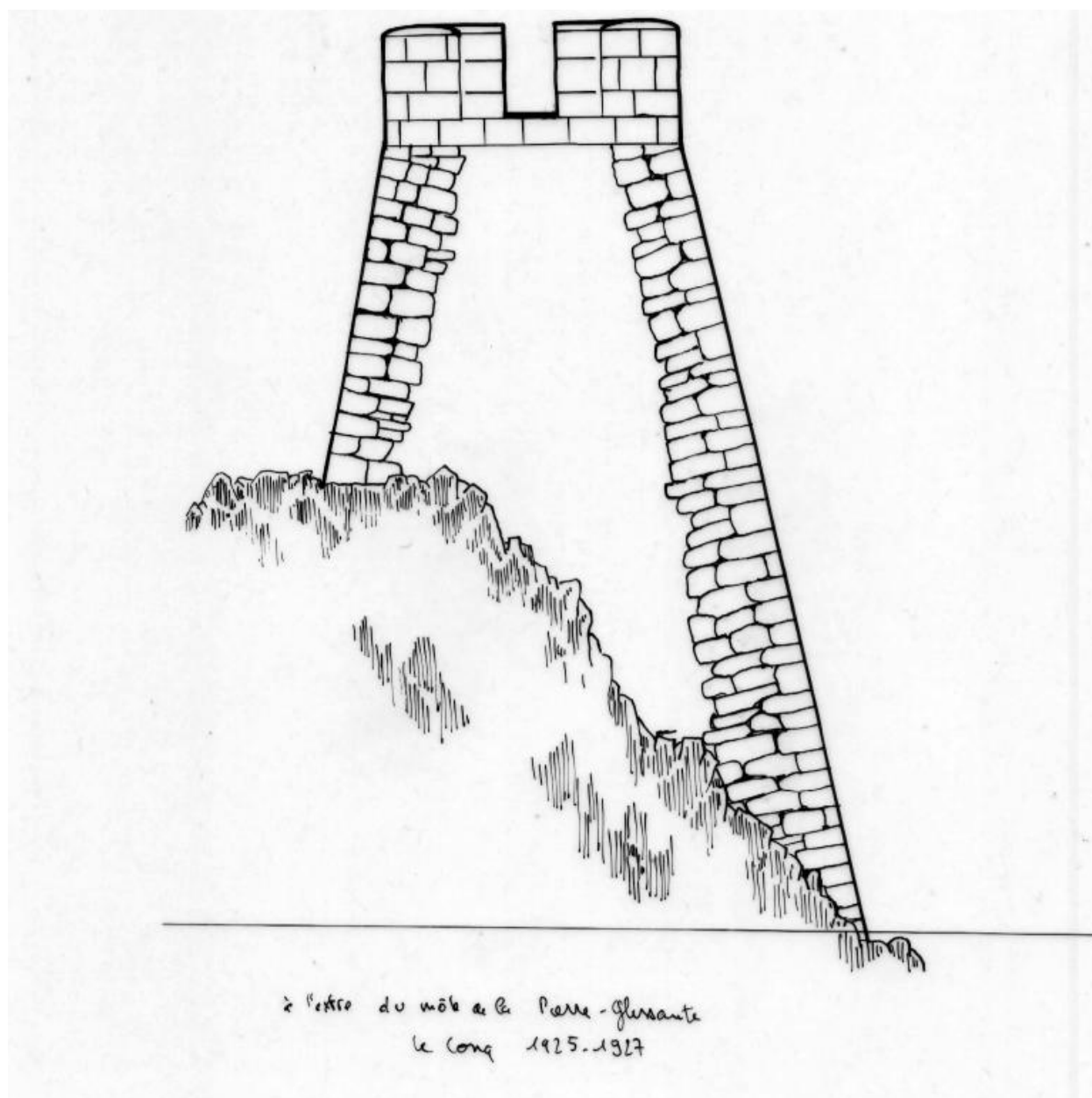
Coupe de la digue de Sainte-Barbe, infrastructure de 1927 (dessin JC Fichou)
