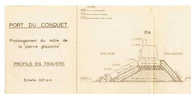
Profil en travers ; Prolongement sur 140m de longueur du môle de la pierre glissante à la pointe de Ste Barbe (30/06/1964 ; projet) Repro. Région Bretagne IVR53_20232905866NUCA
