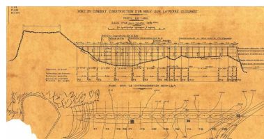
Port du Conquet, construction d'un môle sur la pierre-glissante, profil et plan (1928) Repro. Région Bretagne IVR53_20232905837NUCA
