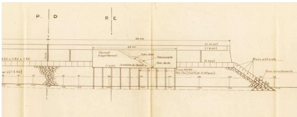
Elévation du prolongement de l'ouvrage (Ponds-et-Chaussées, dressé par l'ingénieur B. Félix, 30/06/64 ; projet)
