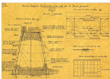
Plan et dessin d'exécution de la construction du môle sur la pierre-glissante (1928) Repro. Région Bretagne IVR53_20232905838NUCA
