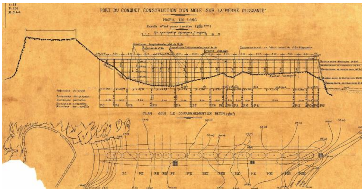
Port du Conquet, construction d'un môle sur la pierre-glissante, profil et plan (1928)
