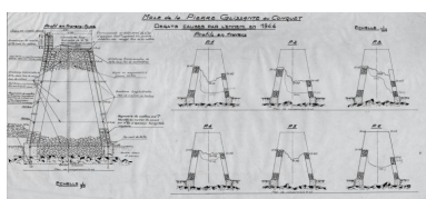
Môle de la pierre-glissante, dégâts causés par l'ennemi en 1944, profil en travers (non daté ; vers 1948) Repro. Région Bretagne IVR53_20232905839NUCB
