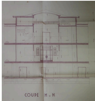
Coupe dans l'axe du chevet. Albert Hec, architecte, 1936. Autr. Albert Hec IVR53_20203505009NUCA
