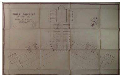
Hospice de vieillards. Plan du premier étage. Albert Hec, architecte, 1936. Autr. Albert Hec IVR53_20203505060A1
