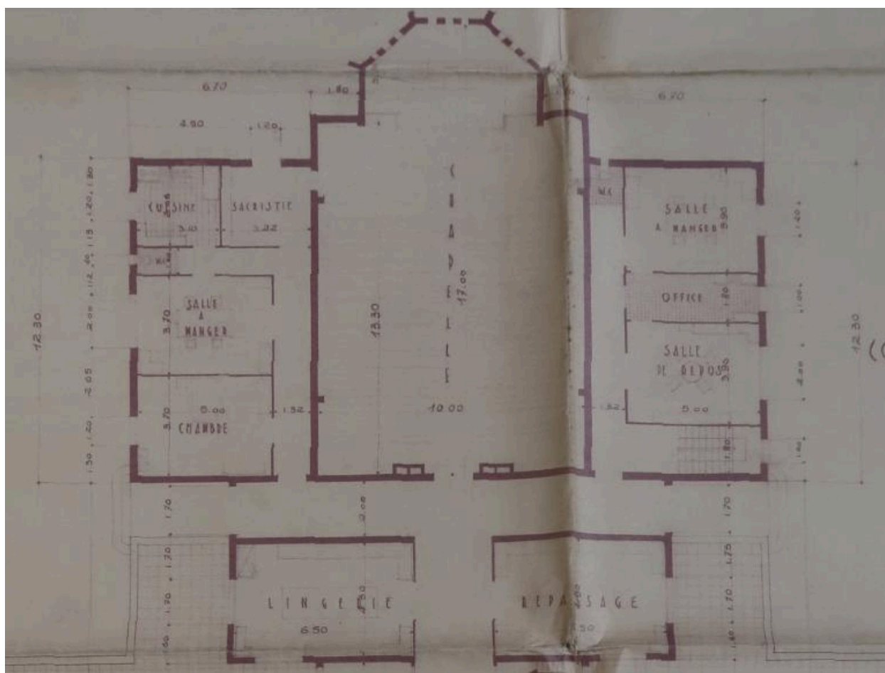
Plan de la chapelle, rez-de-chaussée. Albert Hec, architecte, 1936.
