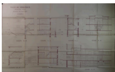
Hospices de vieillards. Coupes. Albert Hec, architecte, 1936.
