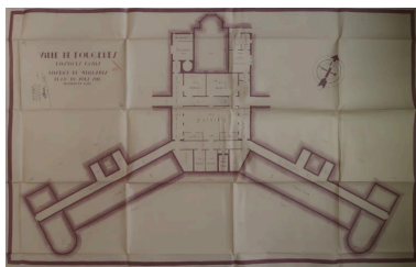
Hospice de vieillards. Plan du sous-sol. Albert Hec, architecte, 1936. Autr. Albert Hec IVR53_20203505062A1
