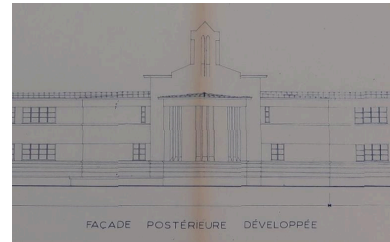
Façades et coupes de l'état existant : détail. Albert Hec et Roger Besnard, architectes, 25/3/1966. Cette élévation est issue de la reconstruction d'après la Seconde Guerre mondiale. Autr. Albert Hec, Autr. Roger Besnard IVR53_20203505082A1
