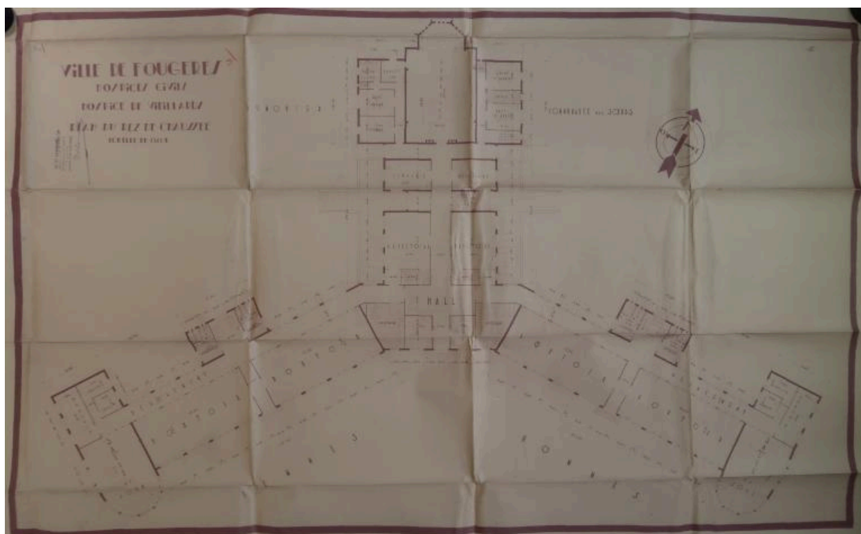
Hospice de vieillards. Plan du rez-de-chaussée. Albert Hec, architecte, 1936.
