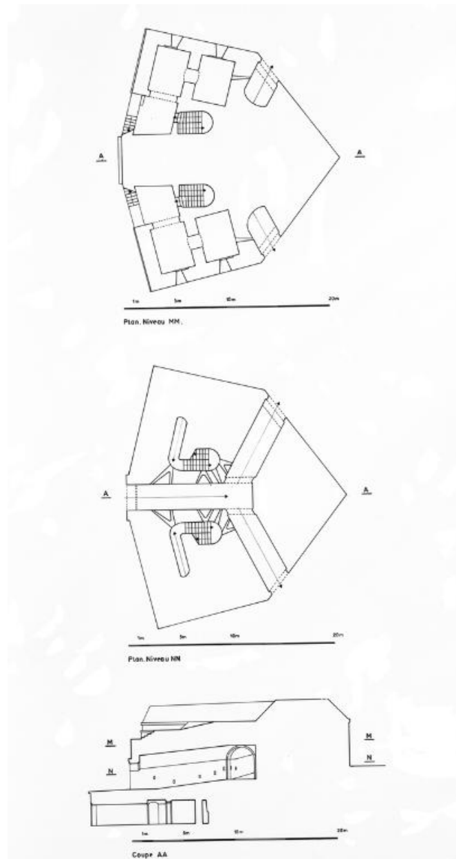
Le Palais, enceinte urbaine, réduit H, plans et coupe.
