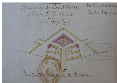
1 VH 286. Place de Belle-Isle, plans, coupes et élévations du réduit en construction de la place d'armes rentrante du front AB indicatif de sa situation au 15 novembre 1809. Phot. Patrick Jadé IVR53_20175608563NUCA
