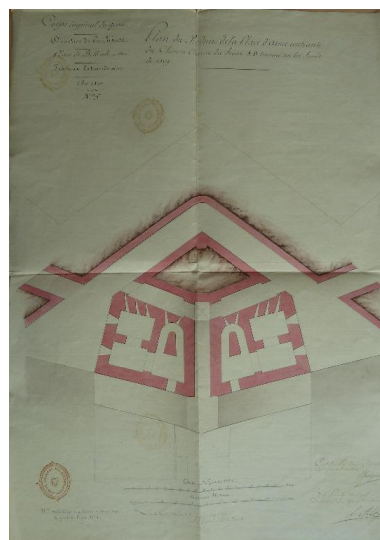
1 VH 286. Place de Belle-Isle, plan du réduit de la place d'armes rentrante du chemin couvert du front AB terminé sur les fonds de 1809, 1810. Phot. Patrick Jadé IVR53_20175608567NUCA
