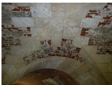
Le Palais, enceinte urbaine, réduit H, grande galerie, carrefour, détail des voûtes. Phot. Patrick Jadé IVR53_20175608592NUCA
