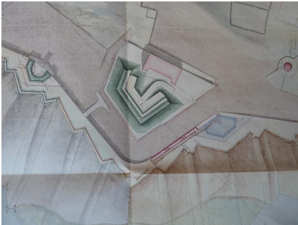
1 VH 286. Place de Belle-île-en-Mer, plan des ouvrages au sud de la citadelle, indicatif de la situation de ces ouvrages à la fin de 1812.
