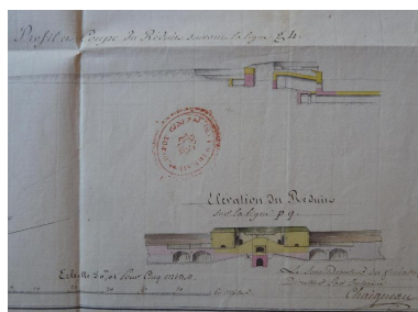
1 VH 286. Place de Belle-Isle, plans, coupes et élévations du réduit en construction de la place d'armes rentrante du front AB indicatif de sa situation au 15 novembre 1809. Phot. Patrick Jadé IVR53_20175608566NUCA
