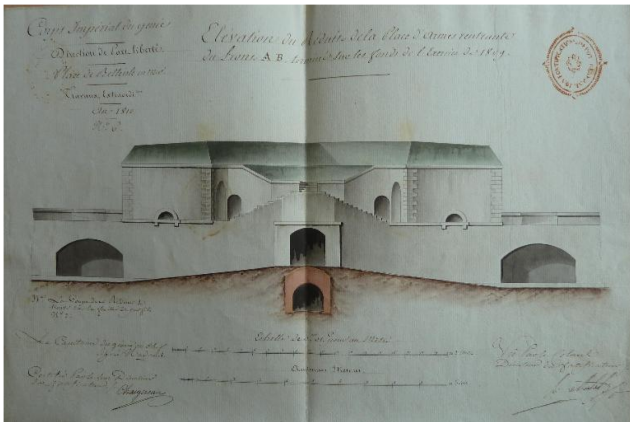
1 VH 286. Place de Belle-Isle, élévation du réduit de la place d'armes rentrante du chemin couvert du front AB terminé sur les fonds de l'exercice 1809, 1810.
