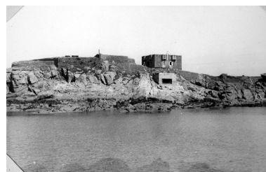
Vue générale de la pointe de Kermorvan : réduit de batterie de côte et casemate-tunnel, n° 81, rapport Pinczon du Sel. Livre IV, vers 1947, Service Historique de la Marine, Brest Phot. Guillaume Lécueillier IVR53_20032901682NUCA
