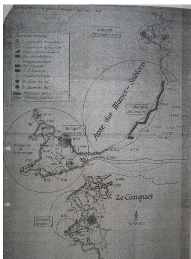
Plan d'ensemble allemand des Stützpunkte Kerlouchouan (Re 38, 39, Re 99-103, Re 124), Le Conquet (Re 40-55), Kermorvan (Re 104-119), Kerlohic (Re 57-58 ; Re 120-123). 5 mars 1943 Phot. Auteur inconnu IVR53_20082910355NUC
