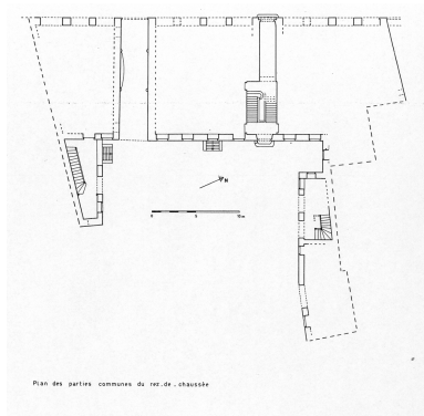
Plan des parties communes du rez-de-chaussée. Phot. Guy Artur, Phot. Norbert Lambart IVR53_19903500074P
