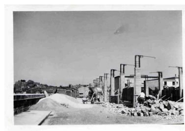
Magasins annexes du Parc en cours de construction (07/06/1949) Phot. Etat IVR53_20232906075NUCB
