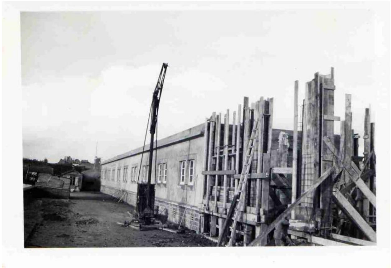
Bâtiment de pilotage en cours de construction (12/1949)
