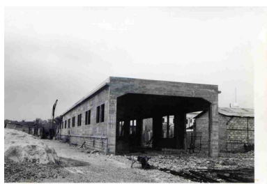
Chantier des magasins en cours (30/07/1949) Phot. Etat IVR53_20232906076NUCB
