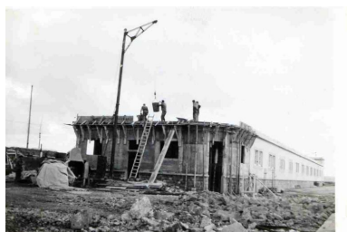
Construction du poste de transformateur en 1951 Phot. Etat IVR53_20232906082NUCB
