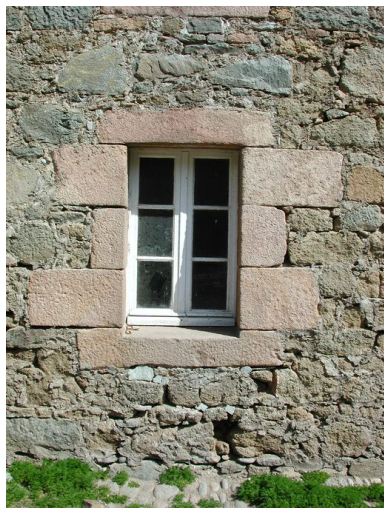
Vue de l'élévation sud : encadrement en pierre de taille de granite rose de l'une des fenêtres (état en 2002) Phot. Guillaume Lécueillier IVR53_20022202488NUCA
