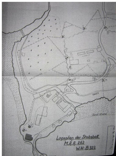
Extrait du plan d'ensemble de la batterie, 1944 (Lageplan der Stabsbatt. M.A.A. 262. W.N. B 323) Phot. Auteur inconnu IVR53_20082910295NUC
