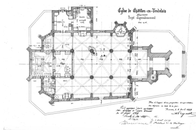
Projet d'agrandissement. Plan au sol. 1899. Autr. Arthur Regnault IVR53_19873500471P
