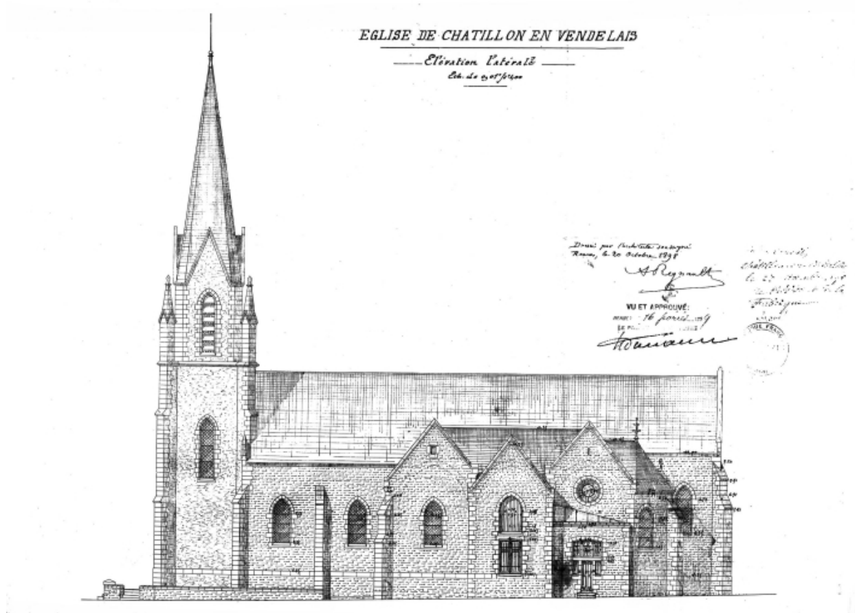
Elévation latérale sud, 1898.
