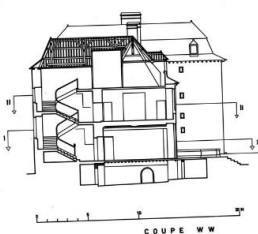
Coupe transversales, partie sud et partie est.
