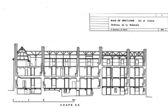
Coupe longitudinale est-ouest.
