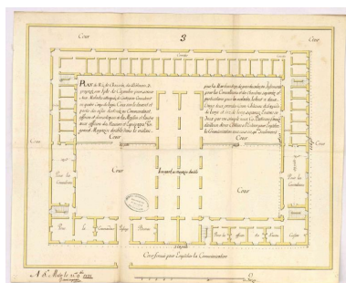
Plan du rez-de-chaussée des logements 3 pour ceux atteints du mal contagieux et magasins pour les marchandises par l'ingénieur Gareneau, 21 septembre 1721. Lavé de couleur jaune, il s'agit d'un projet
