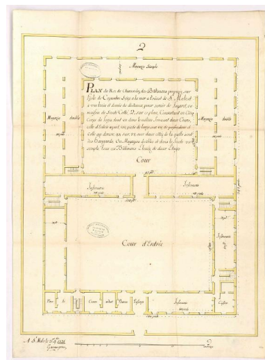
Plan du rez-de-chaussée des bâtiments 2 par l'ingénieur Gareneau, 21 septembre 1721. Lavé de couleur jaune, il s'agit d'un projet Repro. Archives départementales d'Ille-et-Vilaine, Phot. Siméon Gareneau IVR53_20263510336NUCA
