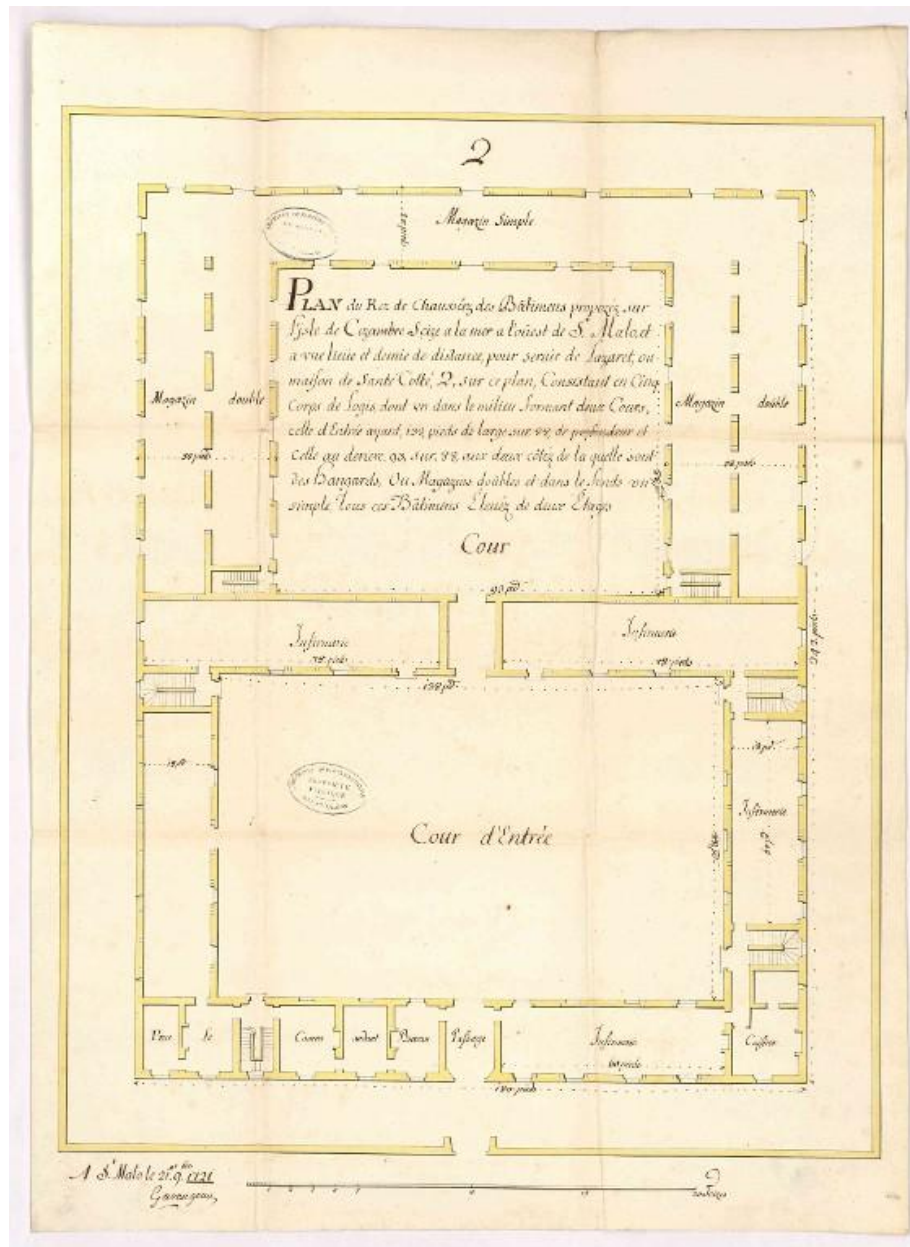
Plan du rez-de-chaussée des bâtiments 2 par l'ingénieur Gareneau, 21 septembre 1721. Lavé de couleur jaune, il s'agit d'un projet
