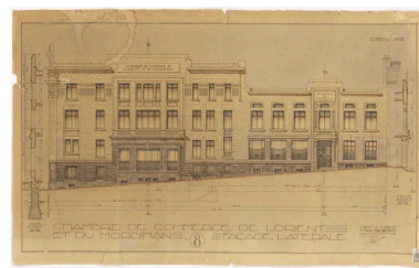
Plan de la façade latérale de la chambre de commerce réalisé en 1927 IVR53_20225605904NUCA
