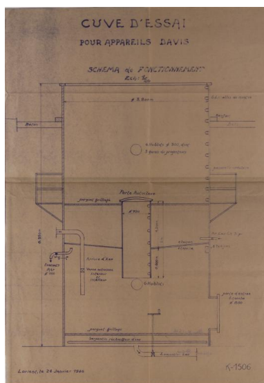
Schéma de fonctionnement de la cuve d'essai pour appareils Davis, plan K n° 1506, 24 janvier 1946 (Service Historique de la Défense de Lorient,
