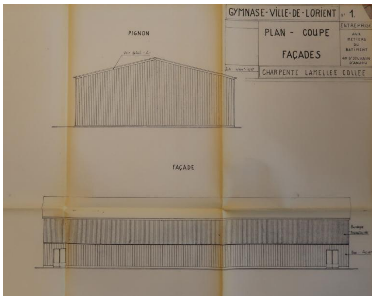
Gymnase Ville de Lorient : plan coupe façades. Entreprise aux métiers du bâtiment, C.O.S.E.C. agréé avec l'architecte Yves Moignet. Sd : vers 1973.
