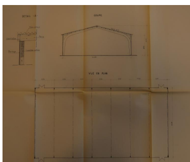
Gymnase Ville de Lorient : plan coupe façades, entreprise aux métiers du bâtiment, C.O.S.E.C. agréé avec l'architecte Yves Moignet. Sd : vers 1973. IVR53_20205605131A0
