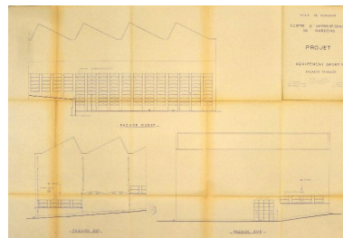
Façades du gymnase, par Y. Moignet et P. Rolland (1956) Phot. Philippe Bonnet IVR53_20172206002NUCA
