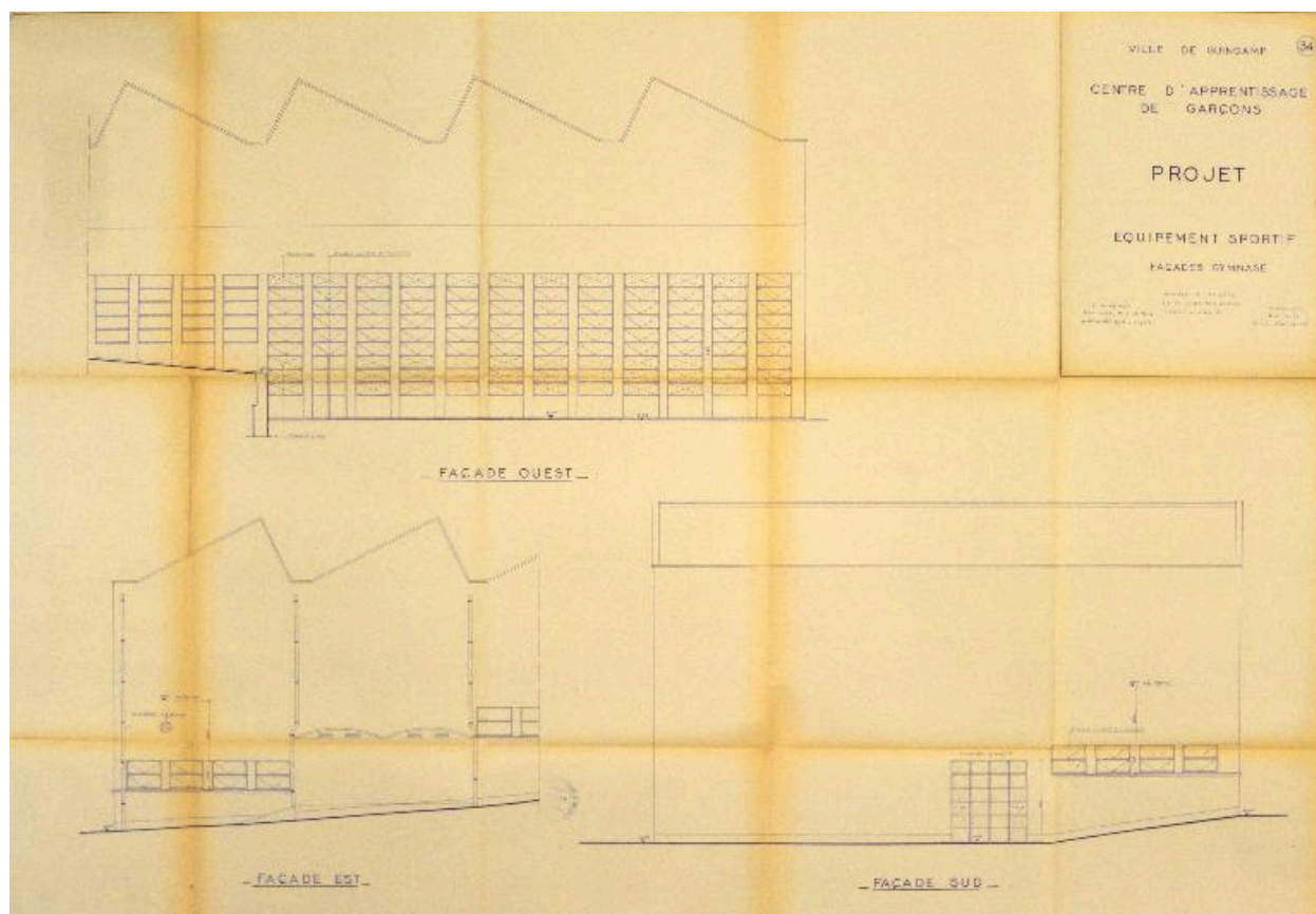
Façades du gymnase, par Y. Moignet et P. Rolland (1956)
