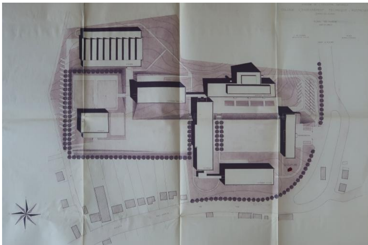
Collège d'enseignement technique de Rostrenen. Plan de masse. 14 décembre 1970. En rouge, l'emplacement projeté de la décoration au titre du 1% artistique. Jean de Jaegher, architecte.
