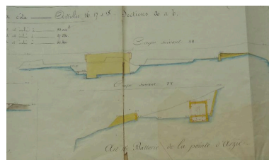
1 VH 294. Place de Belle-Ile, feuille n° 10 des projets extraordinaires pour 1857-1858, 19 février 1857 [papillote de correction du 18 mars 1857].
