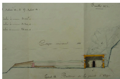
1 VH 296. Place de Belle-Ile, feuille n° 1 des projets pour 1860-1861, 20 novembre 1859. Phot. Patrick Jadé IVR53_20175607151NUCA
