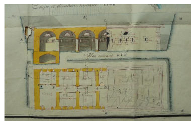
1 VH 296. Place de Belle-Ile, feuille n° 1 des projets pour 1860-1861, 20 novembre 1859.
