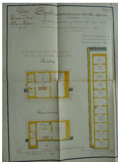
1 VH 294. Place de Belle-Ile, feuille n° 23 des projets extraordinaires pour 1857-1858, détail des modifications apportées aux réduits types, 18 mars 1857. Phot. Patrick Jadé IVR53_20175607152NUCA
