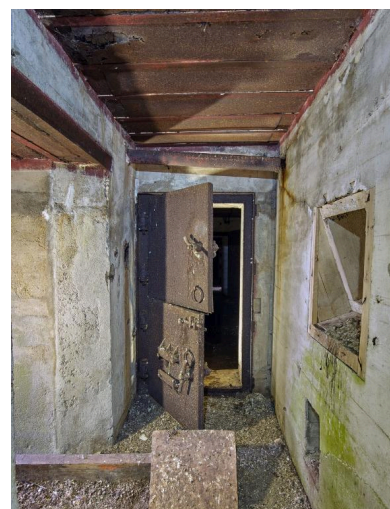
Vue intérieure : porte blindée à deux vantaux du sas. A gauche : couloir d'entrée ouest ; à droite : créneau de défense
