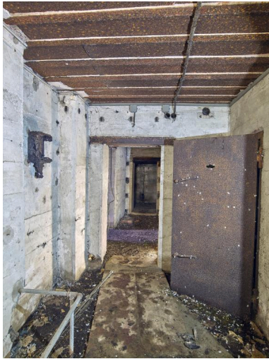
Vue intérieure : couloir du sas et porte étanche. Au fond du couloir, le magasin de munitions est Phot. Bernard Bègne IVR53_20235600226NUCA
