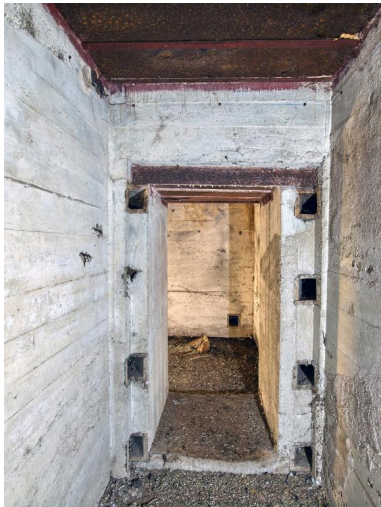
Vue intérieure : emplacement de la porte blindée du magasin de munitions ouest. La porte blindée n'a pas été posée : huit points permettaient de fixer l'hubriserie de la porte Phot. Bernard Bègne IVR53_20235600222NUCA
