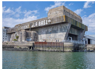
Vue du bunker KI avec l'entrée du slipway : sur la dalle de couverture, le bunker - cuves pour deux canons antiaériens. Sur le quai à gauche, le bunker - casemate de flanquement Phot. Bernard Bègne IVR53_20215600439NUCA
