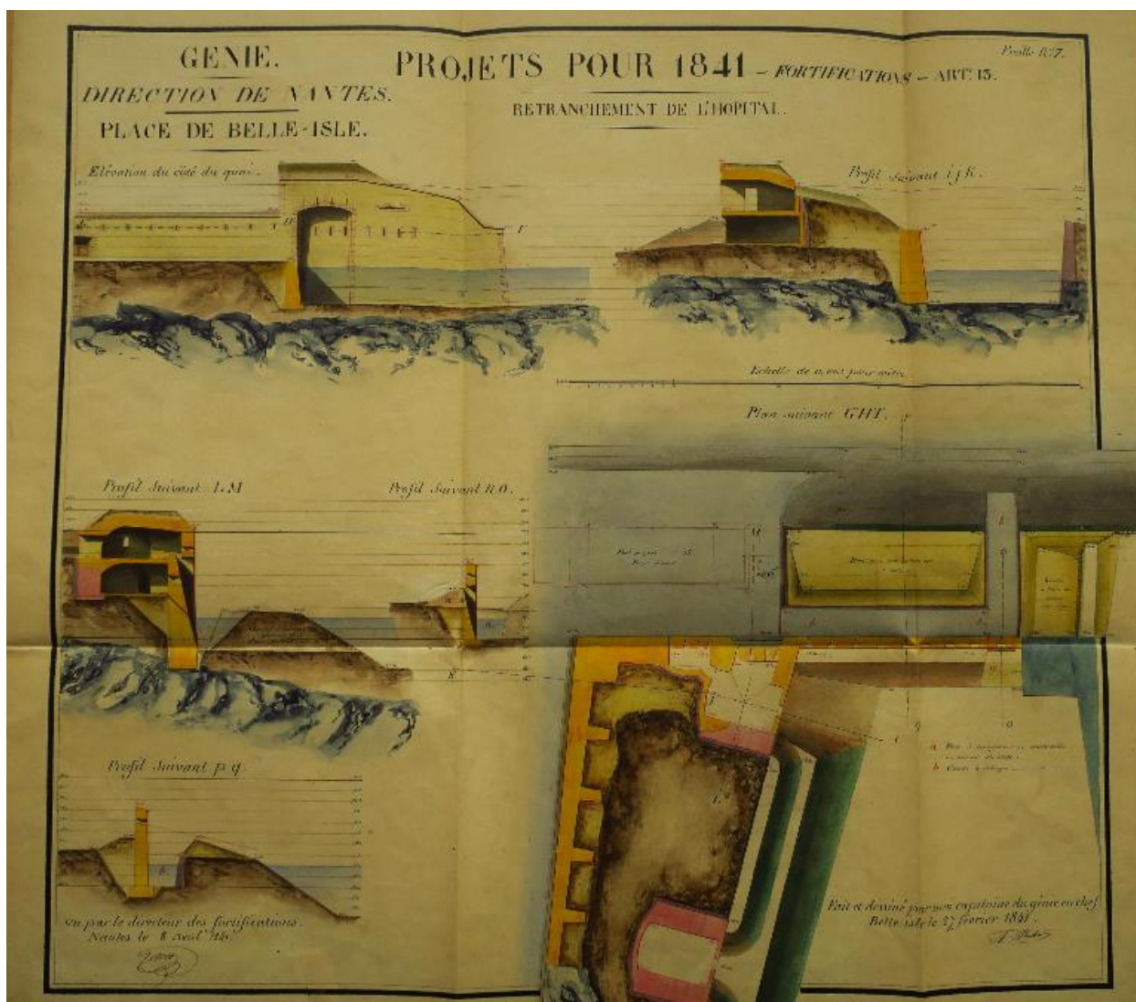
1 VH 290. Place de Belle-Ile, feuille n° 7 des projets pour 1841, retranchement de l'hôpital, 27 février 1841.
