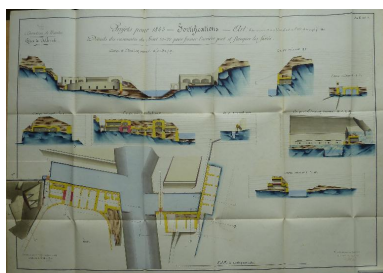
1 VH 291. Place de Belle-Ile, feuille n° 4 des projets pour 1845, détails des casemates du front 21-22 pour fermer l'arrière-port et flanquer les fossés, 16 mars 1845. Phot. Patrick Jadé IVR53_20175608402NUCA
