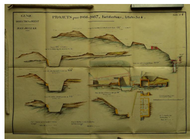
1 VH 297. Place de Belle-Ile, feuille n° 4 des projets pour 1866-1867, courtine 21-22, 7 mars 1866. Phot. Lionel Duigou IVR53_20175608409NUCA
