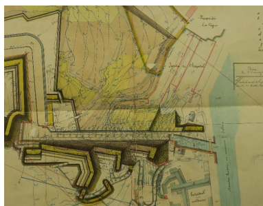
1 VH 297. Place de Belle-Ile, feuille n° 3 des projets pour 1862-1863, bastion 21, courtine 21-22, 2 décembre 1861. Phot. Lionel Duigou IVR53_20175608408NUCA
