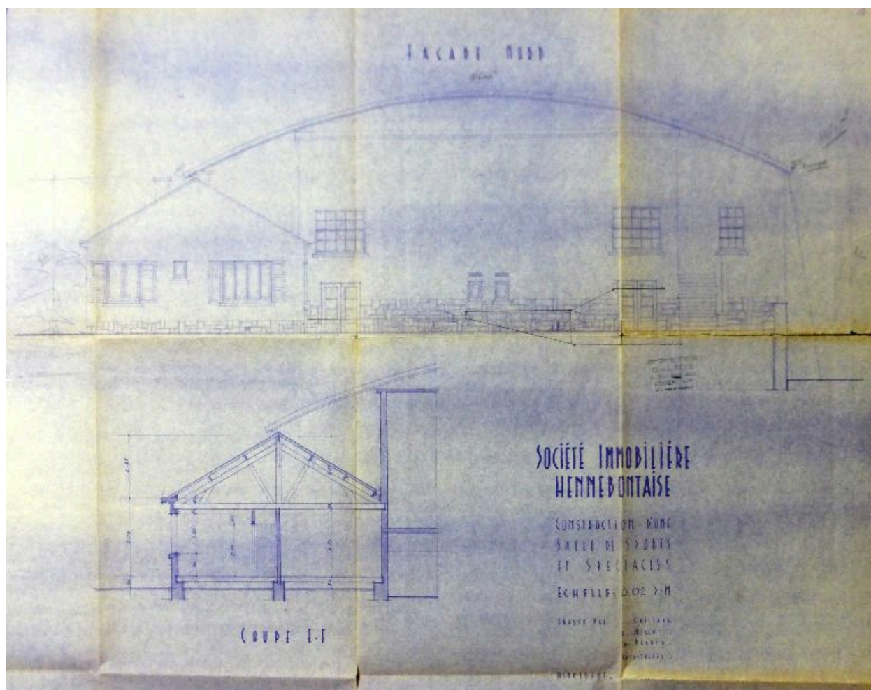
Façade nord et coupe
