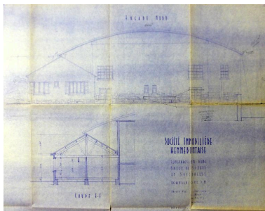
Façade nord et coupe Phot. Philippe Bonnet IVR53_20175606045NUCA
