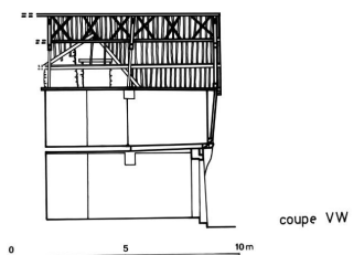
Coupe longitudinale Repro. Guy Artur, Repro. Norbert Lambart, Phot. Auteur inconnu IVR53_19945600045P
