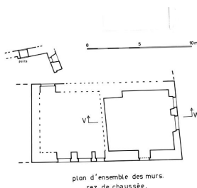
Plan au sol avec le puits Repro. Guy Artur, Repro. Norbert Lambart, Phot. Auteur inconnu IVR53_19945600044P
