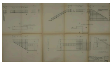
Façade préau. Parement, bacs à fleurs et mur d'about. André Remondet et Patrice Simon, architectes, 15 mars 1961. Une fois encore : le soin du détail. Autr. André Remondet, Autr. Patrice Simon IVR53_20212205035A0
