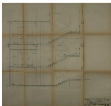
Détail escalier B. Coupe A-B. André Remondet et Patrice Simon, architectes, 7 juillet 1960. Autr. André Remondet, Autr. Patrice Simon IVR53_20212205031A0
