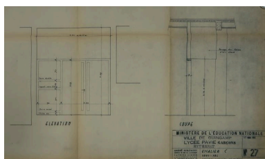
Escalier C, sous-sol. Porte d'accès au préau. André Remondet et Patrice Simon, architectes, 17 mars 1961. Autr. André Remondet, Autr. Patrice Simon IVR53_20212205038A0
