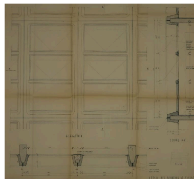
Détail des panneaux de façade. Le principe d'une façade rideau a été retenu. André Remondet et Patrice Simon, architectes, 23 janvier 1959. Autr. André Remondet, Autr. Patrice Simon IVR53_20212205025A0
