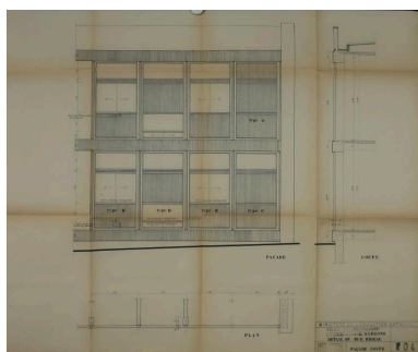
Détail du mur rideau. Façade, coupe, plan. André Remondet et Patrice Simon, architectes, 25 juillet 1960. Autr. André Remondet, Autr. Patrice Simon IVR53_20212205029A0
