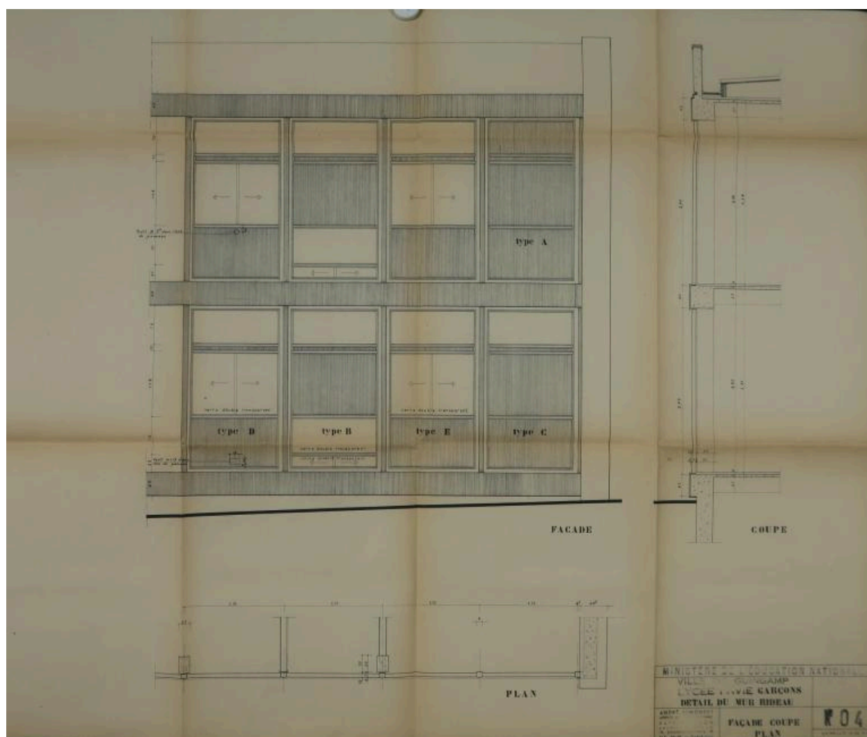
Détail du mur rideau. Façade, coupe, plan. André Remondet et Patrice Simon, architectes, 25 juillet 1960.
