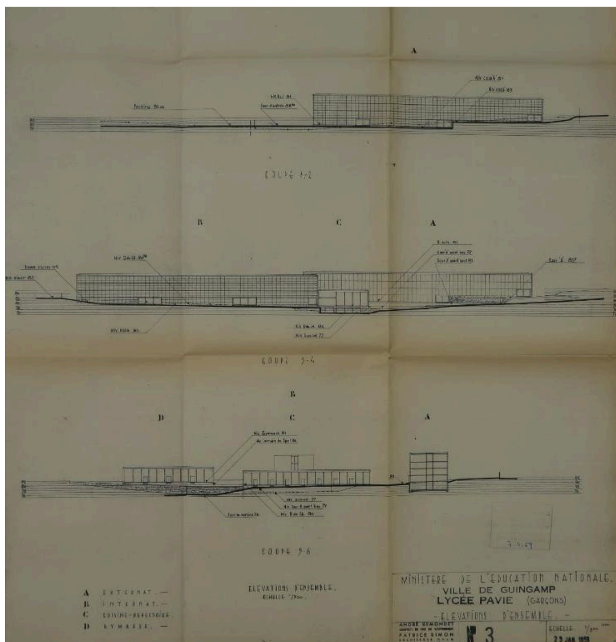
Élévations d'ensemble. André Remondet et Patrice Simon, architectes, 23 janvier 1959.
