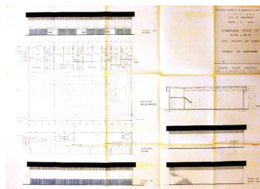
Plans, coupe, façades, par J.-C. Le Bail & J. Penven, 1967 Phot. Philippe Bonnet IVR53_20162905535NUCA
