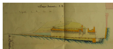
1 VH 293. Place de Belle-Ile, feuille n° 1 des projets pour 1849, 25 mai 1849. Phot. Lionel Duigou IVR53_20175608058NUCA
