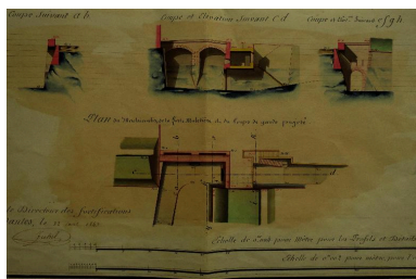
1 VH 291. Place de Belle-Ile, feuille n° 3 des projets pour 1843, escarpement de la côte, pour fermer la place entre le port et l'extrémité de la coupure 18, 29 mars 1843.
