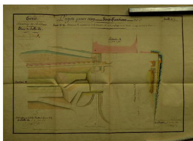
1 VH 293. Place de Belle-Ile, feuille n° 1 des projets pour 1849, 25 mai 1849. Phot. Lionel Duigou IVR53_20175608056NUCA
