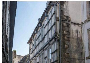
Des lisses hautes et basses filent sur l'étage, lequel est contreventé par des poteaux et écharpes. Phot. Charlotte Barraud IVR53_20252900589NUCA
