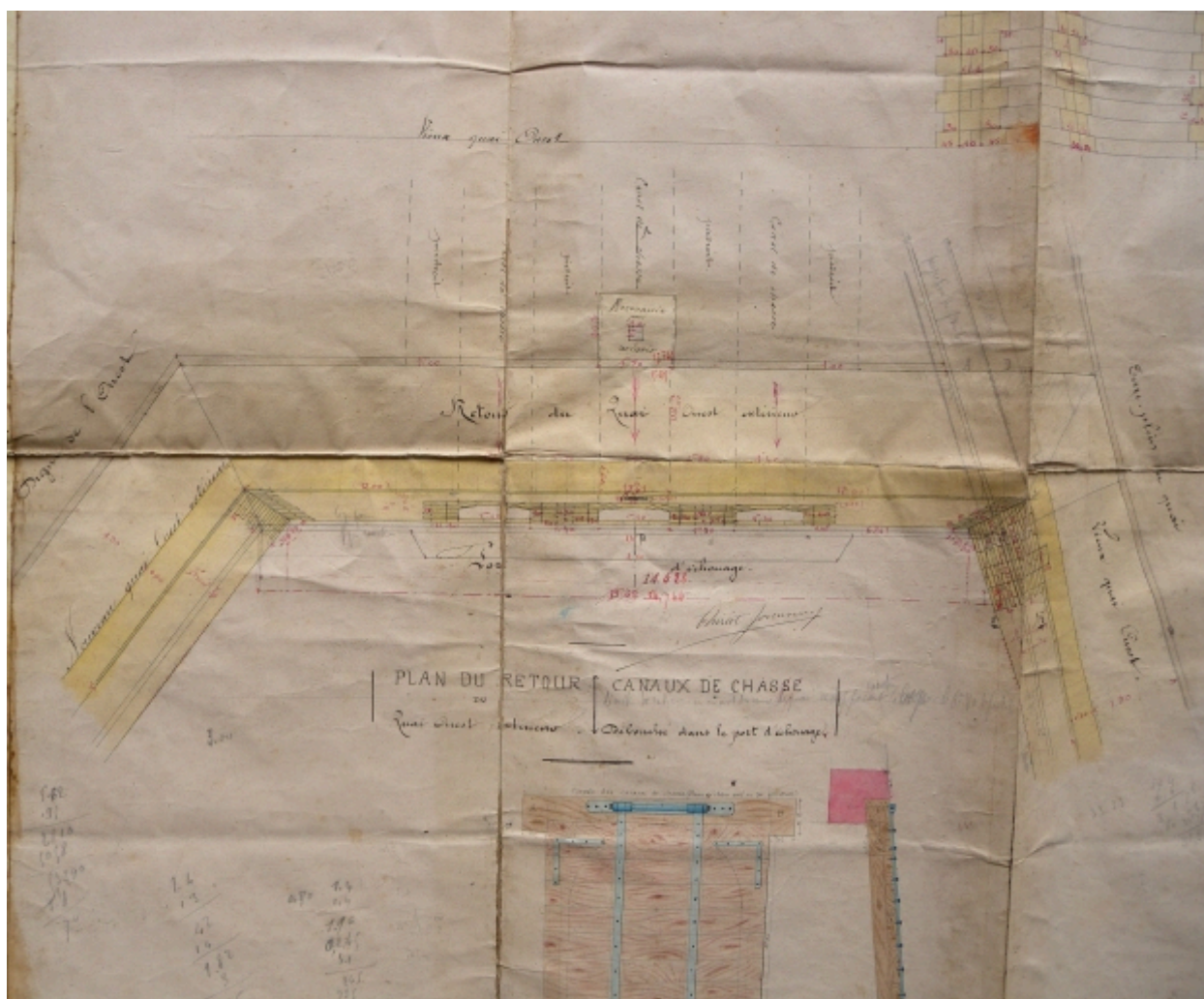
Plan de retour des canaux de chasse, 1882 (AD 22)
