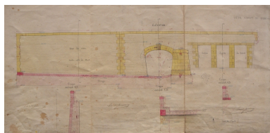
Plan : élévation et coupe de l'aqueduc du Quinic, 1882 (AD 22) Phot. Guy Prigent, Autr. Jourjon IVR53_20092212410NUCB
