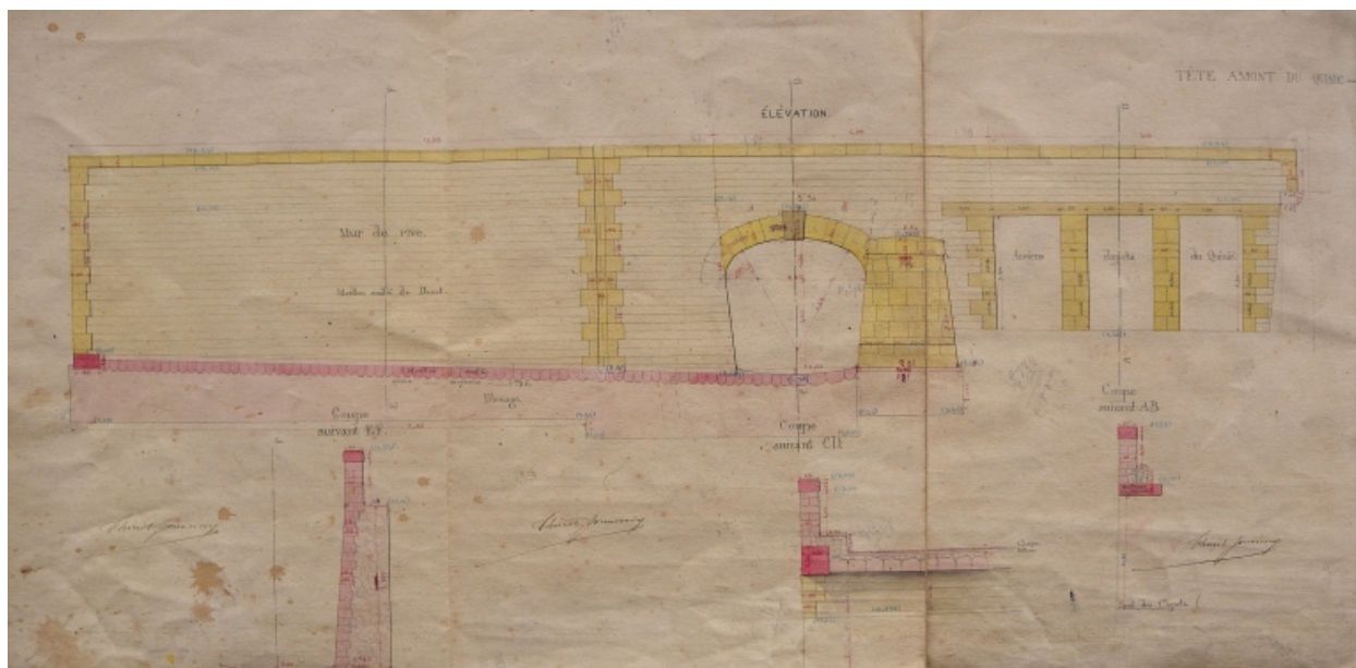
Plan : élévation et coupe de l'aqueduc du Quinic, 1882 (AD 22)
