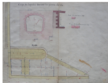
Plan : coupe de l'aqueduc du Quinic, 1882 (AD 22) Phot. Guy Prigent, Autr. Jourjon IVR53_20092212411NUCB
