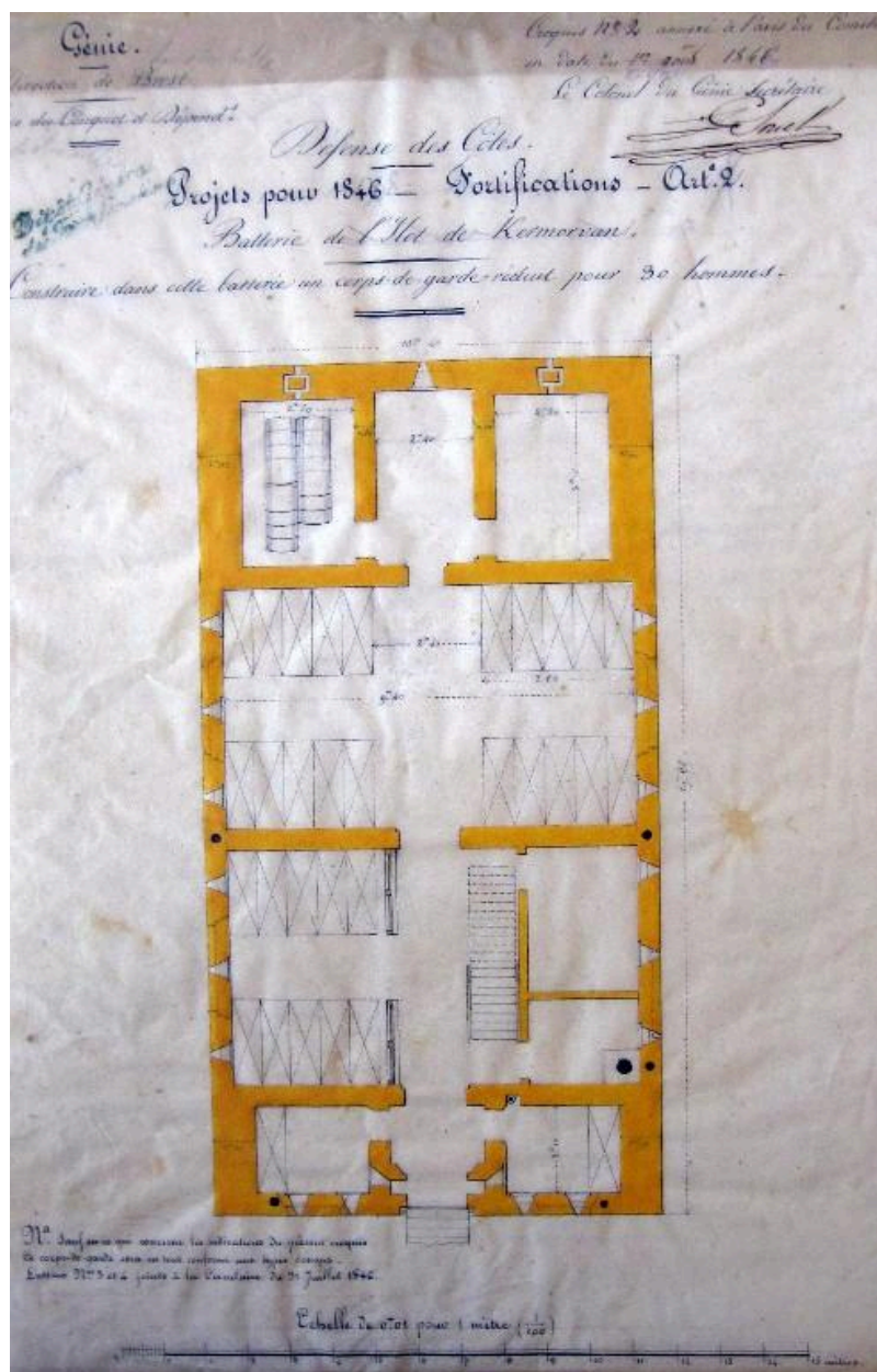
Plan du corps de garde crénelé pour 30 hommes pour la batterie de l'Îlette de Kermorvan, projet pour 1846
