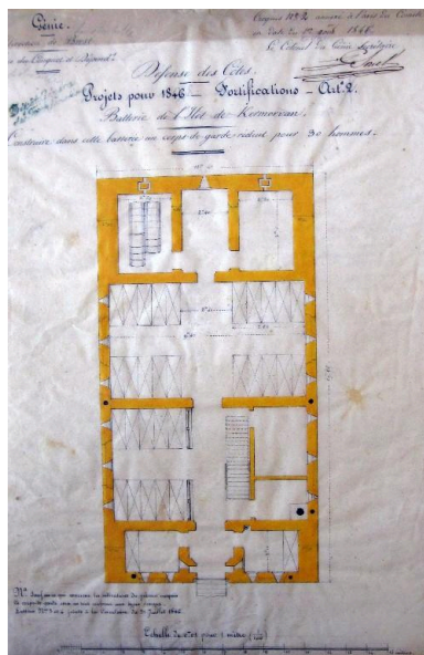
Plan du corps de garde crénelé pour 30 hommes pour la batterie de l'Îlet de Kermorvan, projet pour 1846 Phot. Patrick Jadé IVR53_20242910018NUCA
