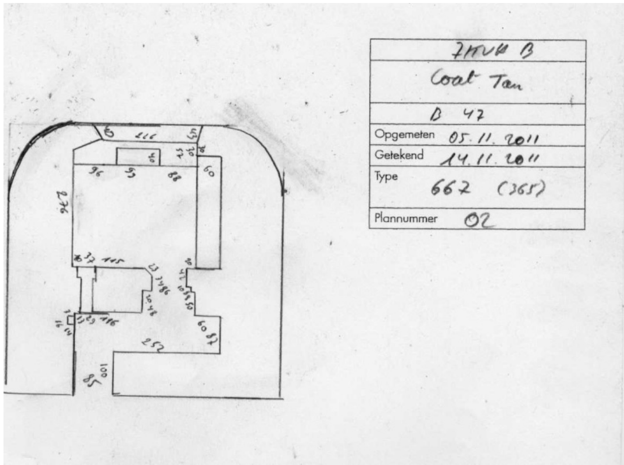
Plan du bunker - casemate de type 667 (365) (dessin : Dirk Peeters)
