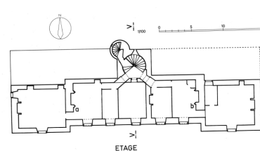
Plan à l'étage
