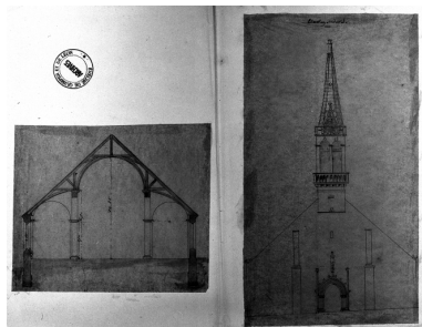
Châteaulin, église paroissiale Saint-Idunet : Elévation et coupe, Joseph Bigot, 1867. (A.E. Quimper) Phot. François Dagorn IVR53_19682900044V
