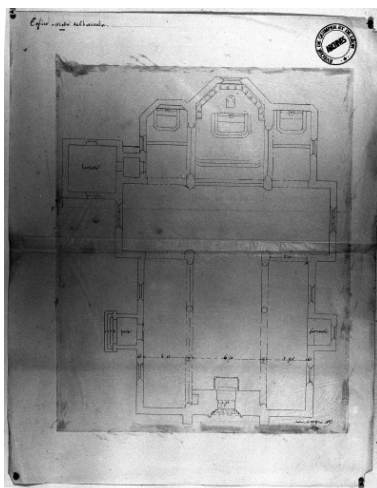
Châteaulin, église paroissiale Saint-Idunet : Plan au sol, Joseph Bigot, 1867 (A.E. Quimper). Phot. François Dagorn IVR53_19682900043V
