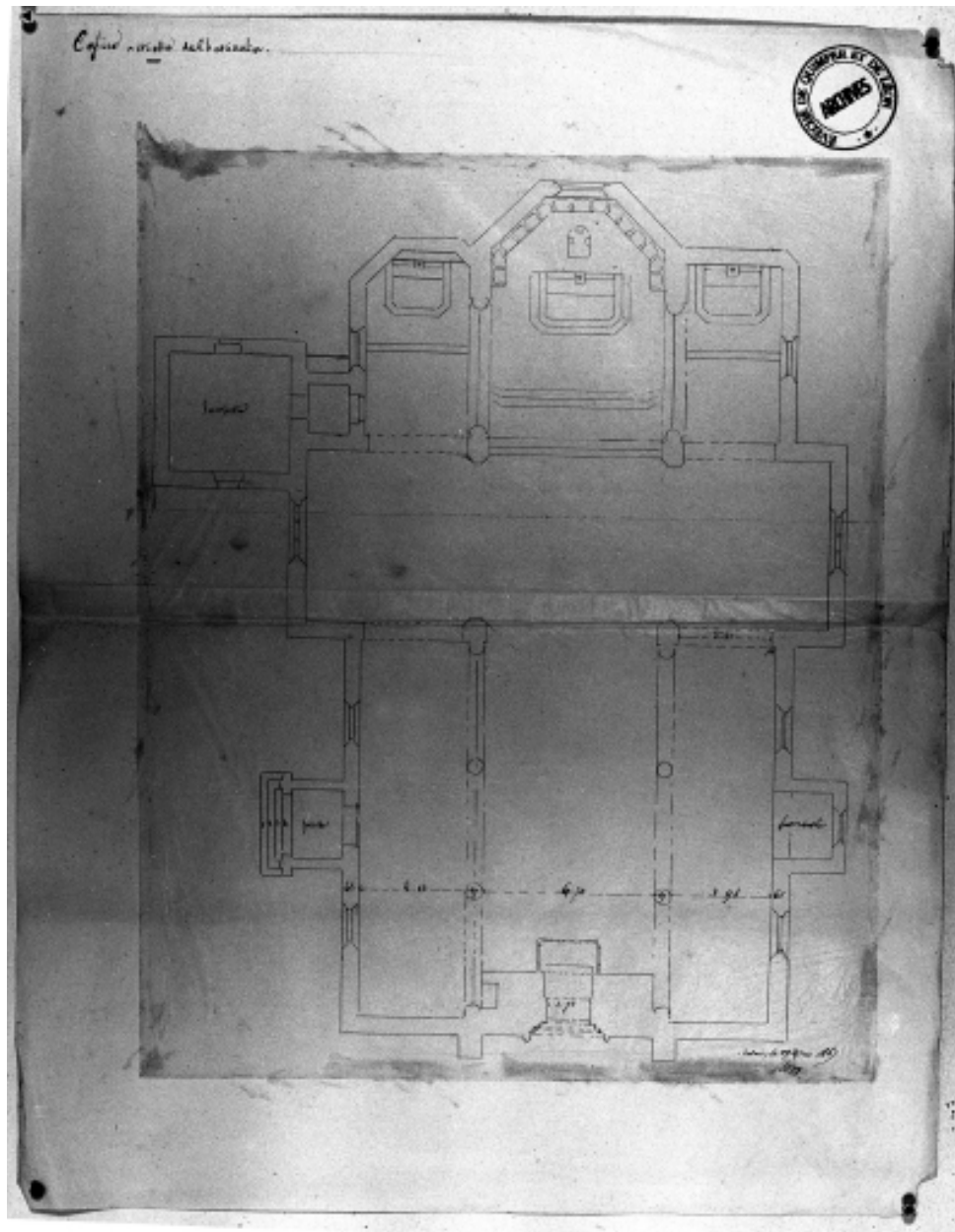
Châteaulin, église paroissiale Saint-Idunet : Plan au sol, Josph Bigot, 1867 (A.E. Quimper).
