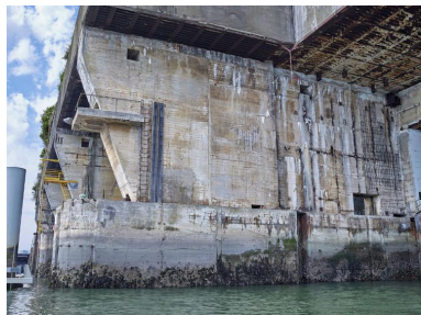
Vue de l'entrée de l'alvéole F (n° 15 et 16) : contrefort du mur latéral Phot. Bernard Bègne IVR53_20215600520NUCA
