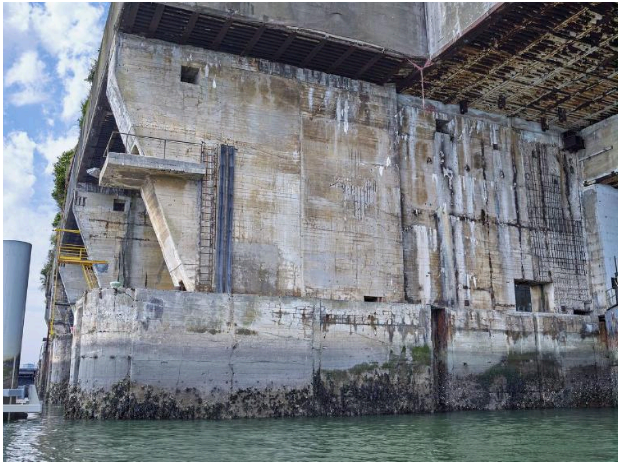
Vue de l'entrée de l'alcôve F (n° 15 et 16) : contrefort du mur latéral
