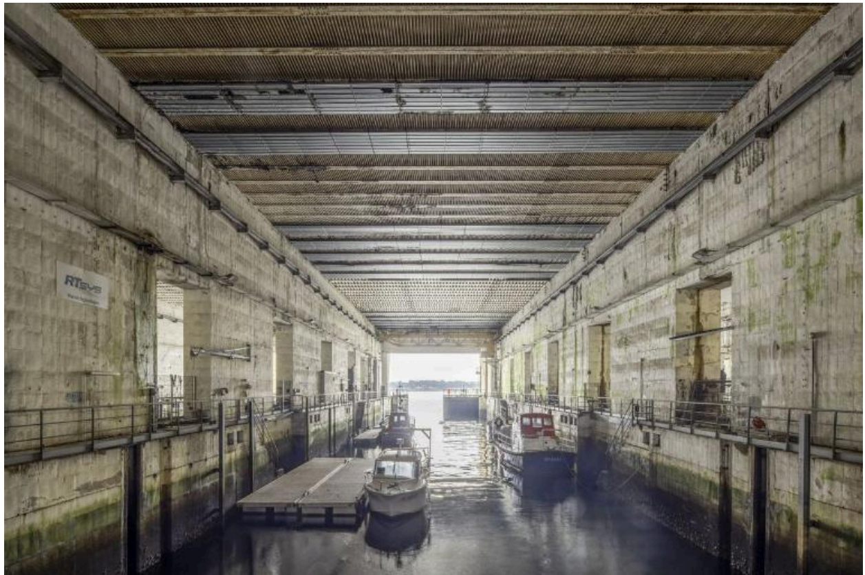
Vue générale de l'alvéole F (n° 15 et 16) en eau depuis la "rue"
