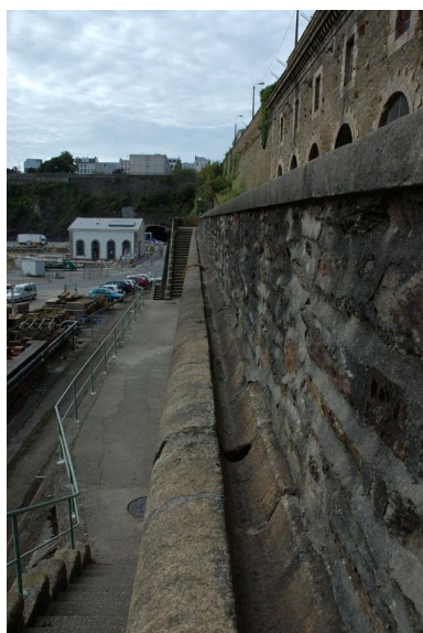
Vue de détail : rigole en granite destinée à collecter les eaux pluviales de la chaussée - terrasse supérieure Phot. Guillaume Lécueillier IVR53_20072906735NUCA
