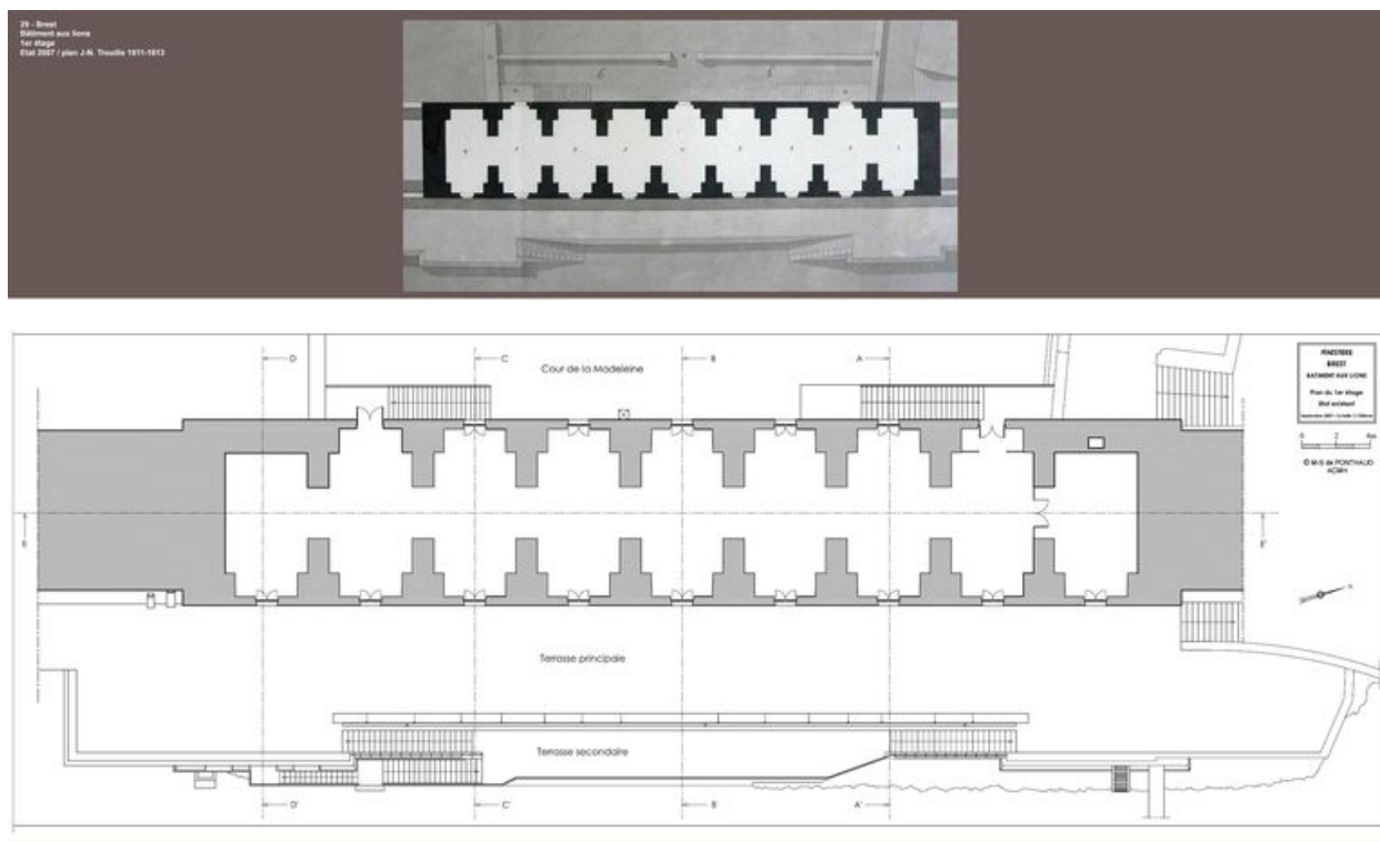
Plan du 1er étage, état existant, septembre 2007. Plan de Jean-Nicolas Trouille, 1811-1813 (extrait de l'étude préalable à la restauration de Marie-Suzanne de Ponthaud, Architecte en Chef des Monuments Historiques)
