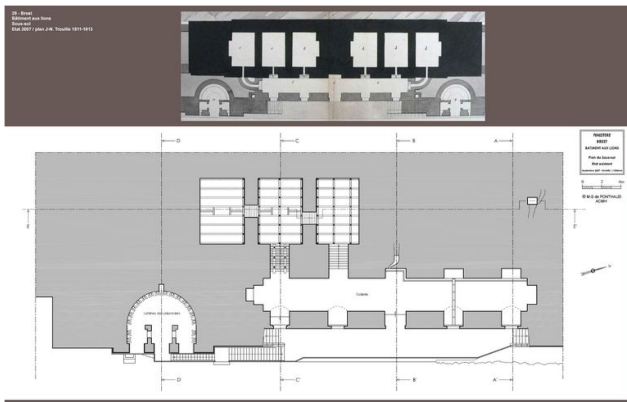
Plan du sous-sol, état existant, septembre 2007. Plan de Jean-Nicolas Trouille, 1811-1813 (extrait de l'étude préalable à la restauration de Marie-Suzanne de Ponthaud, Architecte en Chef des Monuments Historiques)
