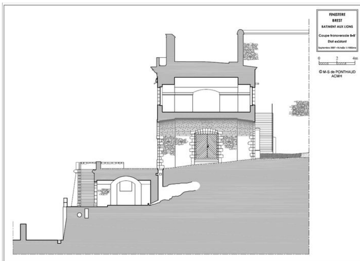
Coupe transversale B-B', état existant, septembre 2007 (extrait de l'étude préalable à la restauration de Marie-Suzanne de Ponthaud, Architecte en Chef des Monuments Historiques)
