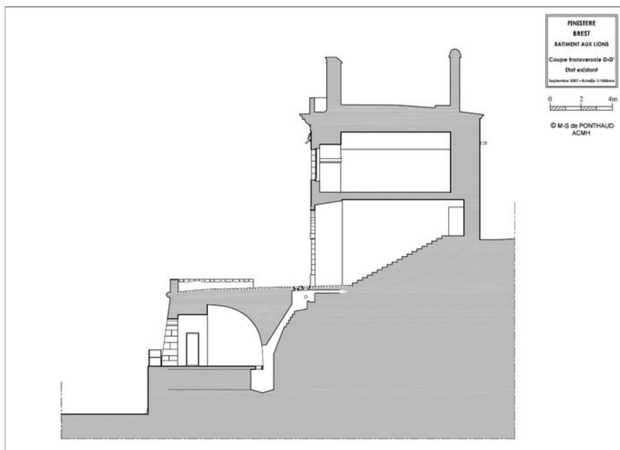
Coupe transversale D-D', état existant, septembre 2007 (extrait de l'étude préalable à la restauration de Marie-Suzanne de Ponthaud, Architecte en Chef des Monuments Historiques)
