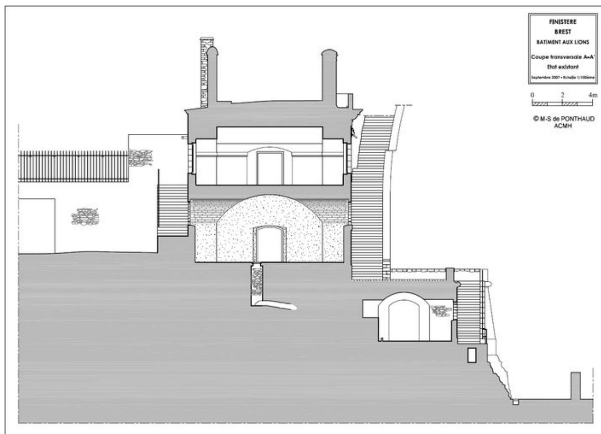
Coupe transversale A-A', état existant, septembre 2007 (extrait de l'étude préalable à la restauration de Marie-Suzanne de Ponthaud, Architecte en Chef des Monuments Historiques)
