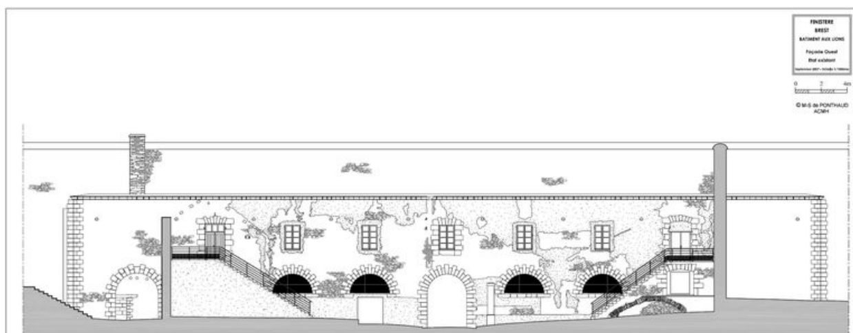
Élévation ouest, état existant, septembre 2007 (extrait de l'étude préalable à la restauration de Marie-Suzanne de Ponthaud, Architecte en Chef des Monuments Historiques)
