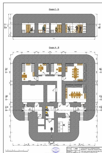
Plan et coupe d'un bunker-poste de direction de tir de type L 404 pour batterie antiaérienne lourde (Unterstand mit Befehls Stand, schwere Flak) Dess. Christian Moigneux IVR53_20263510110NUCA
