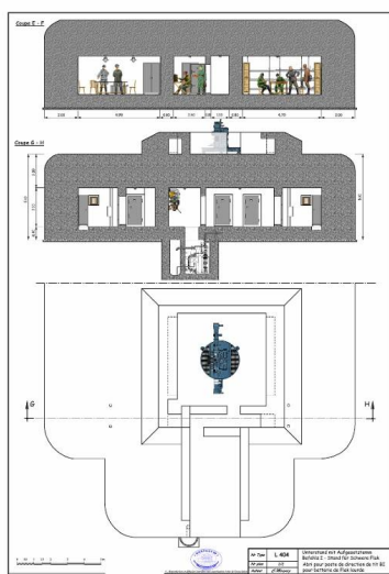
Plan et coupes d'un bunker-poste de direction de tir de type L 404 pour batterie antiaérienne lourde (Unterstand mit Befehls Stand, schwere Flak) Dess. Christian Moigneux IVR53_20263510111NUDA
