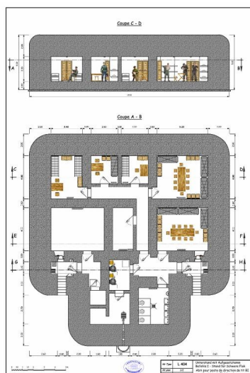
Plan et coupe d'un bunker-poste de direction de tir de type L 404 pour batterie antiaérienne lourde (Unterstand mit Befehls Stand, schwere Flak) Dess. Christian Moigneux IVR53_20263510111NUDA
