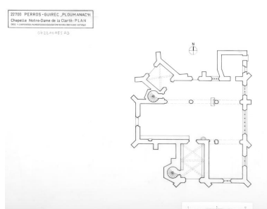
Plan au sol Dess. Yves Carpentier IVR53_20072210185A3
