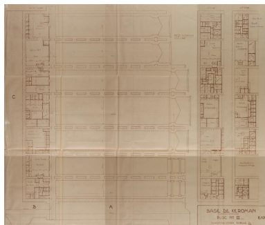
Plan d'ensemble du bunker KIII : bassins et locaux, plan K n ° 5, 11 décembre 1945 (Service Historique de la Défense de Lorient, Monographie de la base Ingénieur Général Stosskopf, 1945-1946) Phot. Service Historique de la Défense IVR53_20235605304NUCA
