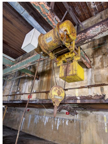
Vue de l'extension nord-ouest : détail du treuil d'une capacité de 3 tonnes au troisième étage Phot. Bègne Bernard IVR53_20235600753NUCA
