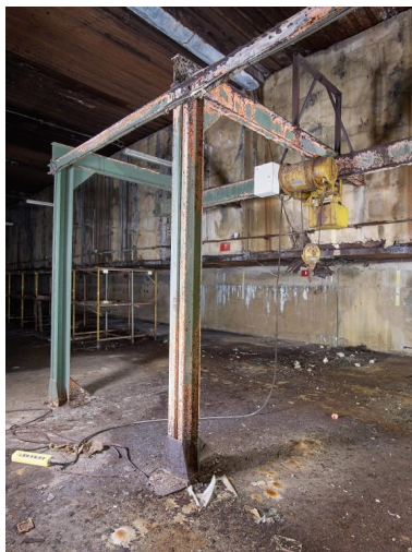
Vue de l'extension nord-ouest : potence et treuil d'une capacité de 3 tonnes au troisième étage Phot. Bègne Bernard IVR53_20235600752NUCA
