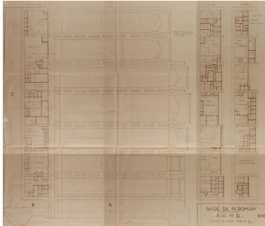
Plan d'ensemble du bunker KIII : bassins et locaux, plan K n° 5, 11 décembre 1945 (Service Historique de la Défense de Lorient, Monographie de la base Ingénieur Général Stosskopf, 1945-1946) Phot. Service Historique de la Défense IVR53_20235605304NUCA
