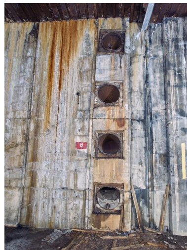
Vue de l'extension nord-ouest : tuyaux du système de ventilation traversant le mur nord-ouest au troisième étage Phot. Bègne Bernard IVR53_20235600754NUCA
