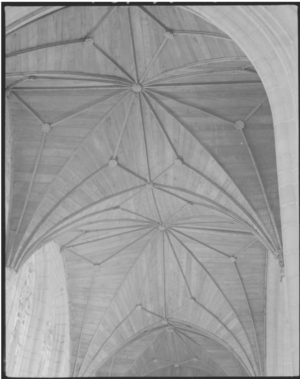
Couvrement du bas-côté sud
