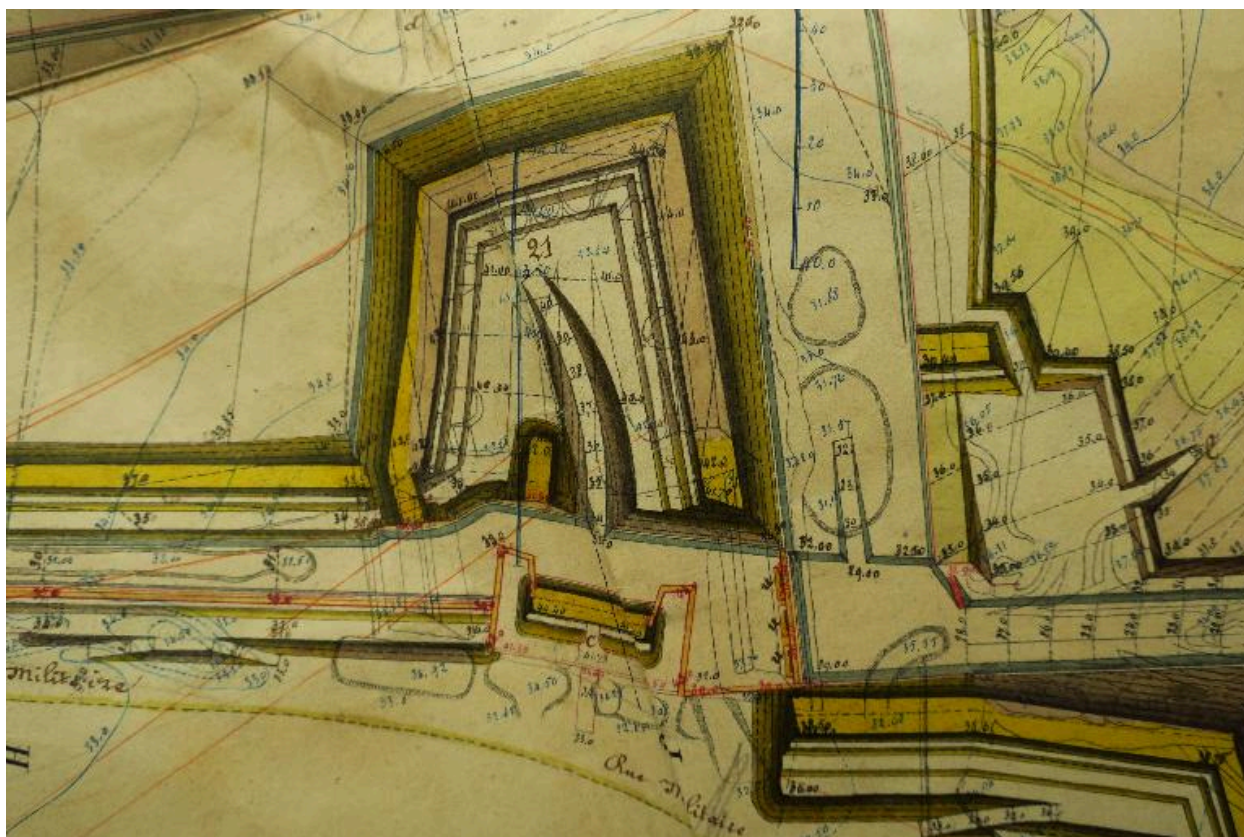
1 VH 296. Place de Belle-Ile, feuille n° 8 des projets pour 1860-1861, 14 juillet 1860.
