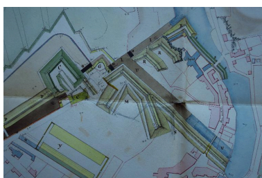
1 VH 289. Place de Belle-Isle-en-Mer, feuille n° 1 des projets pour 1831, projet d'ensemble pour la place de Palais, 1er mars 1831.
