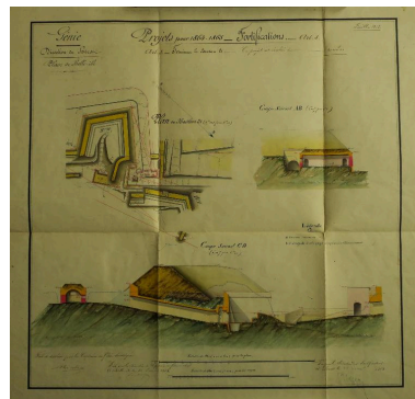
1 VH 297. Place de Belle- Ile, feuille n° 2 des projets pour 1864-1865, terminer le bastion 21, 30 janvier 1864. Phot. Lionel Duigou IVR53_20175608345NUCA
