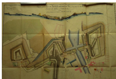
1 VH 291. Place de Belle-Ile, feuille n° 4 des projets pour 1843, enceinte de Palais, front 21-22, 29 mars 1843.
