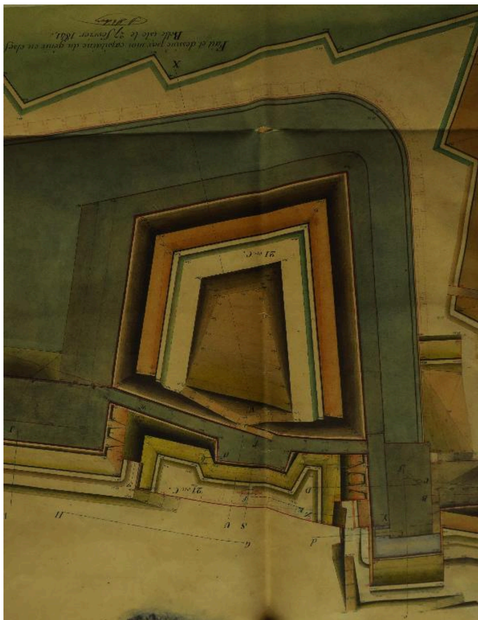
1 VH 290. Place de Belle-Ile, feuille n° 5 des projets pour 1841, achèvement de l'enceinte de Palais, 27 février 1841.
