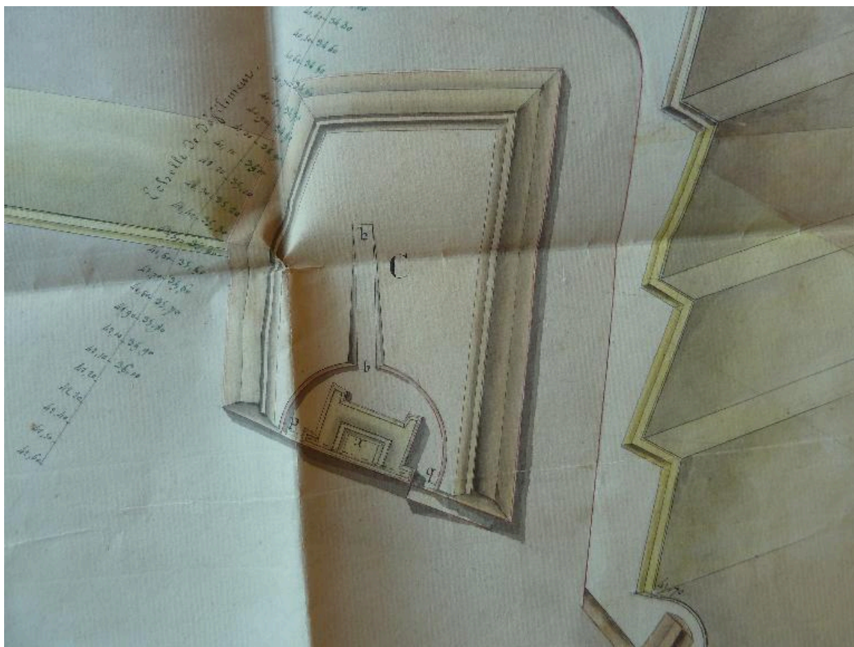
1 VH 286. Place de Belle-île-en-Mer, nouveau projet de fortifications entreprises sur le plateau au sud de la citadelle, 1809.
