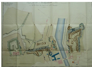
1 VH 291. Place de Belle-Ile, feuille n° 5 des projets pour 1845, état des lieux du front 21-22 ou C et Beausoleil, 16 août 1843.
