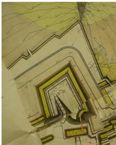
1 VH 297. Place de Belle- Ile, feuille n° 3 des projets pour 1862-1863, bastion 21, courtine 21-22, 2 décembre 1861. Phot. Lionel Duigou IVR53_20175608344NUCA
