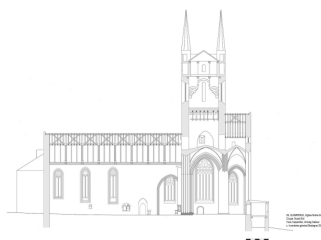
Coupe longitudinale
