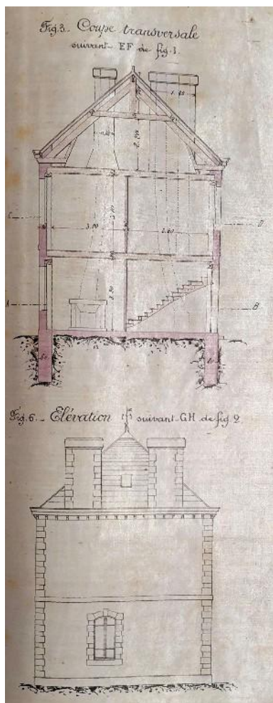
Plans de l'avant-projet de construction de logements pour le maître de port
