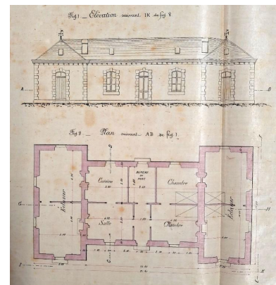
Projet de construction de logement pour le maître de port et les éclusières, étude avec simple rez-de-chaussée (24 avril 1888) Repro. Erwana L'Haridon IVR53_20262210130NUCA
