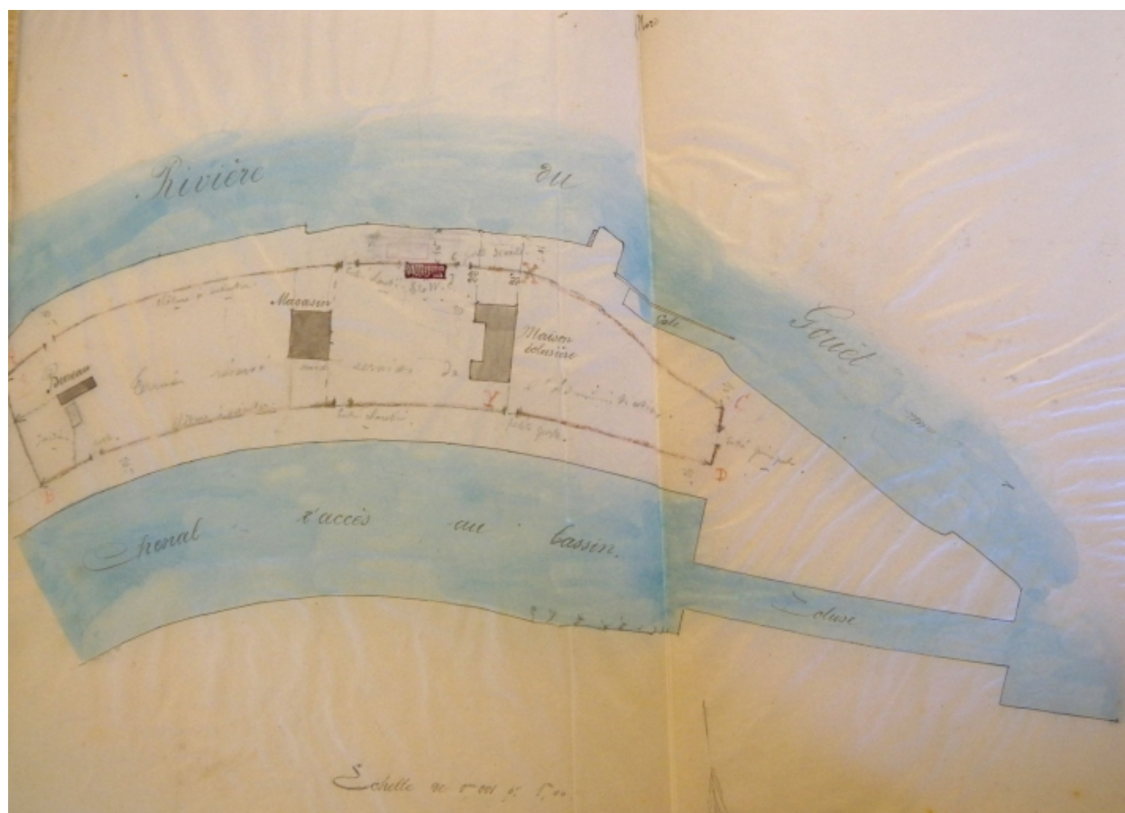
Plan : emplacement de la maison éclusière, du bureau et du magasin, 1892 (Ad 22)
