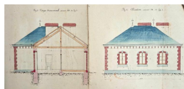
Projet de construction de logement pour le maître de port et les éclusiers (9 octobre 1888) Repro. Erwana L'Haridon IVR53_20262210128NUCA
