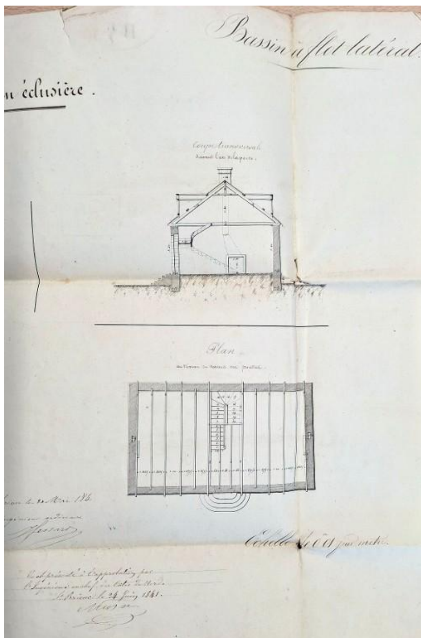
Maison éclusière, plan dressé par le service des Ponts-et-Chaussées (30 mai 1841)
