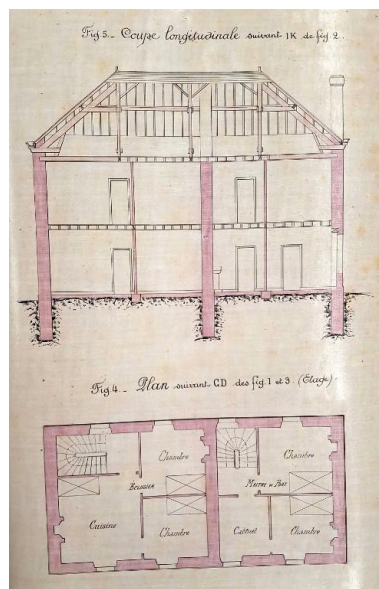
Plans de l'avant-projet de construction de logements pour le maître de port et les éclusiers, étude avec rez-de- chaussées et étage (24 avril 1888) Repro. Erwana L'Haridon IVR53_20262210133NUCA
