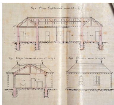
Projet de construction de logement pour le maître de port et les éclusiers, étude avec simple rez-de-chaussée (24 avril 1888) Repro. Erwana L'Haridon IVR53_20262210131NUCA
