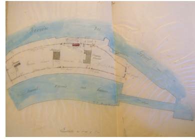
Plan : emplacement de la maison éclusière, du bureau et du magasin, 1892 (Ad 22) Repro. Guy Prigent, Phot. Auteur inconnu IVR53_20082213170NUCB
