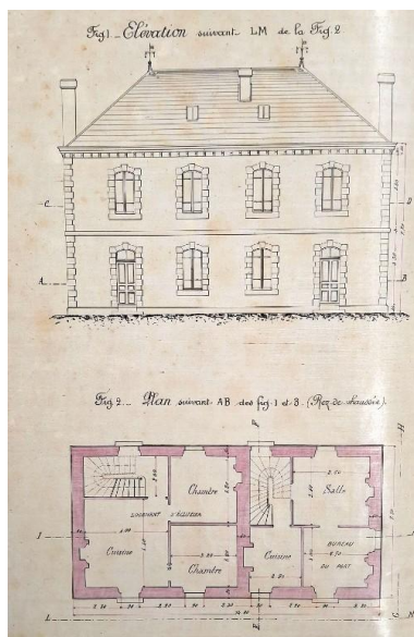
Plans de l'avant-projet de construction de logements pour le maître de port et les éclusiers, étude avec rez-de- chaussées et étage (24 avril 1888) Repro. Erwana L'Haridon IVR53_20262210132NUCA
