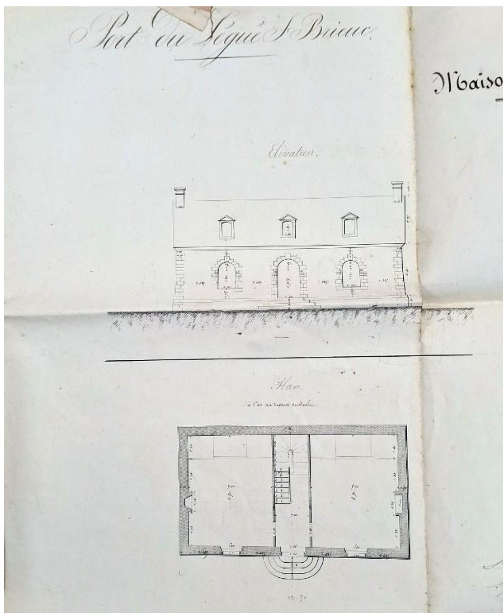
Maison éclusière, plan dressé par le service des Ponts-et-Chaussées (30 mai 1841)
