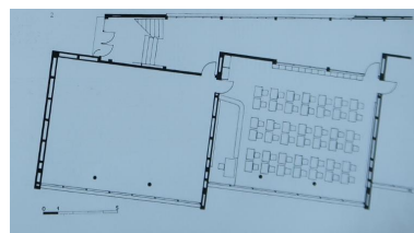
Plan partiel du bâtiment des classes (extrémité ouest du bâtiment), in Rambert [Charles], Constructions scolaires et universitaires, pp. 104-107. Autr. Lopez Raymond IVR53_20252910028NUC
