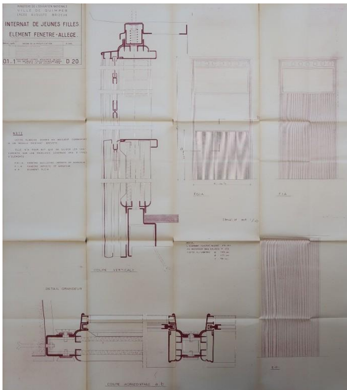
Internat de jeunes filles. Elément fenêtre allège. Raymond Lopez, architecte, 1952.
