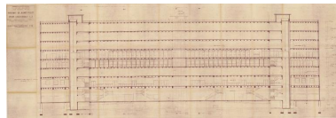
Internat de jeunes filles. Coupe longitudinale. Raymond Lopez, architecte, 1952. Autr. Raymond Lopez IVR53_20252910009A0
