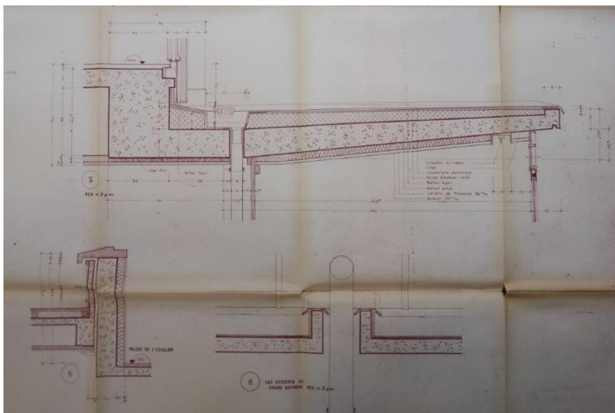
Internat de jeunes filles. Détails des toitures (vue partielle du plan). Raymond Lopez, architecte, 1952.
