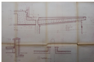
Internat de jeunes filles. Détails des toitures (vue partielle du plan). Raymond Lopez, architecte, 1952. Autr. Raymond Lopez IVR53_20252910011A0
