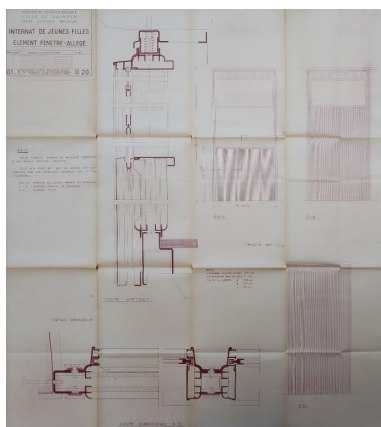
Internat de jeunes filles. Élément fenêtre allège. Raymond Lopez, architecte, 1952. Autr. Raymond Lopez IVR53_20252910019A0
