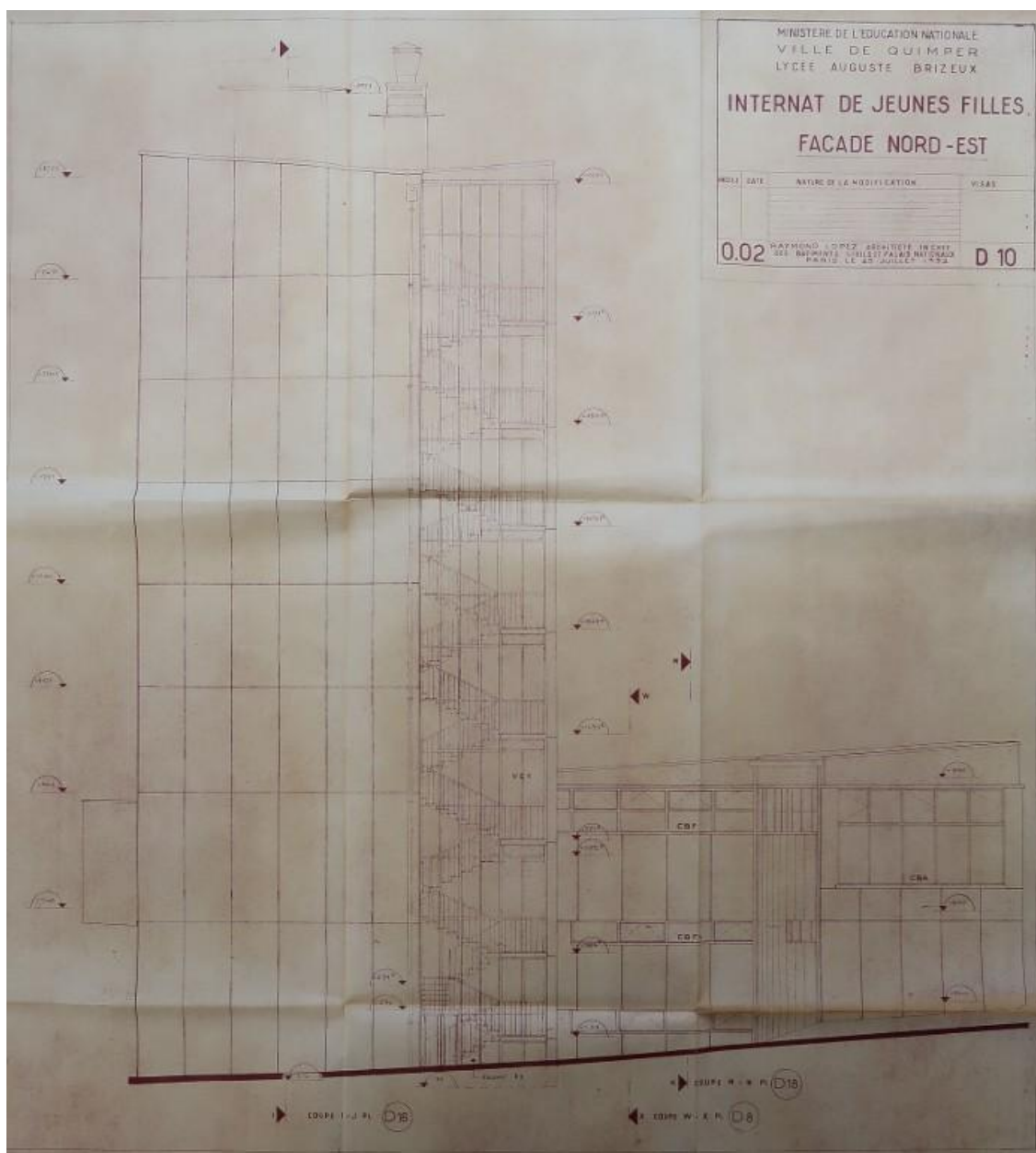
Internat de jeunes filles. Façade nord-est. Raymond Lopez, architecte, 1952.
