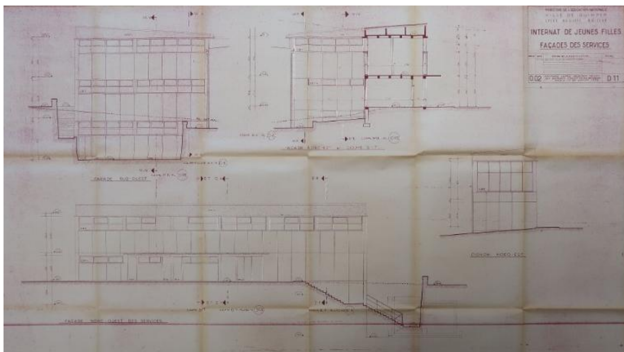
Internat de jeunes filles. Façade des services. Raymond Lopez, architecte, 1952.
