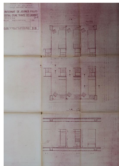
Internat de jeunes filles. Détail d'une travée de cabines. Raymond Lopez, architecte, 1952. Autr. Raymond Lopez IVR53_20252910018A0
