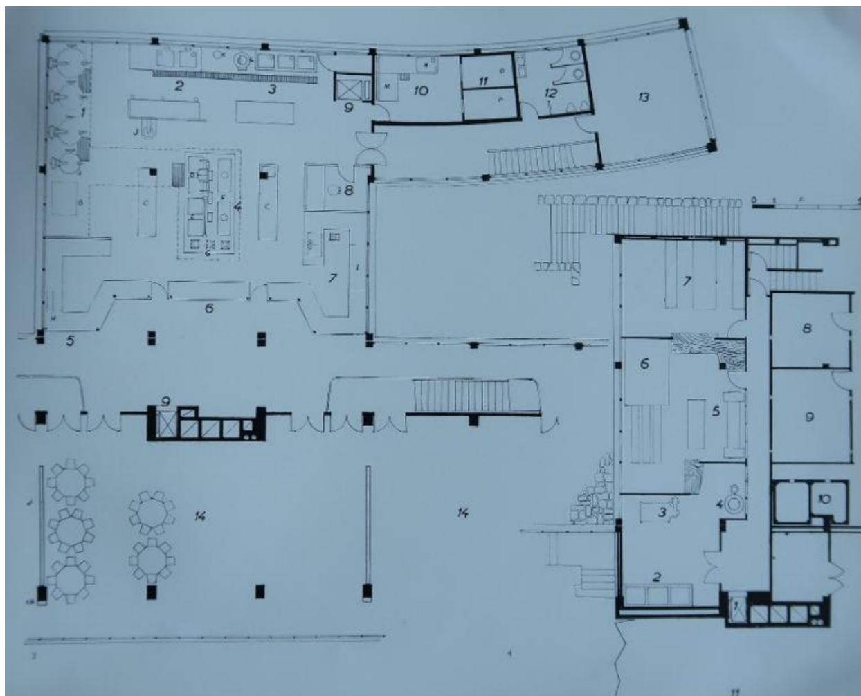
Plan des cuisines et d'une salle de réfectoire. In Rambert [Charles], Constructions scolaires et universitaires , pp. 104-107.
