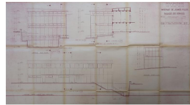
Internat de jeunes filles. Façade des services. Raymond Lopez, architecte, 1952. Autr. Raymond Lopez IVR53_20252910014A0
