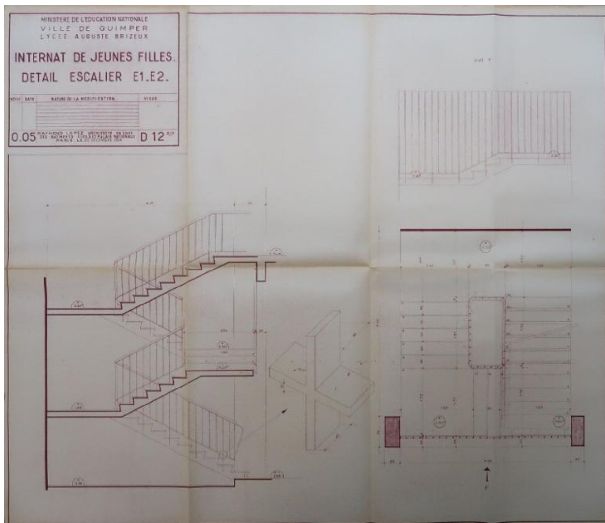
Internat de jeunes filles. Détail escalier E1 - E2. Raymond Lopez, architecte, 1952.
