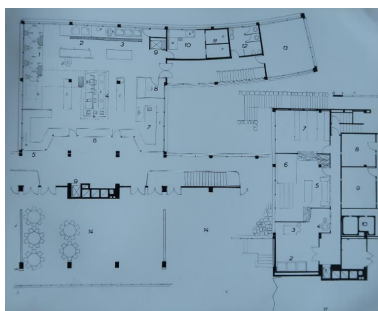
Plan des cuisines et d'une salle de réfectoire. In Rambert [Charles], Constructions scolaires et universitaires, pp. 104-107. Autr. Lopez Raymond IVR53_20252910025NUC
