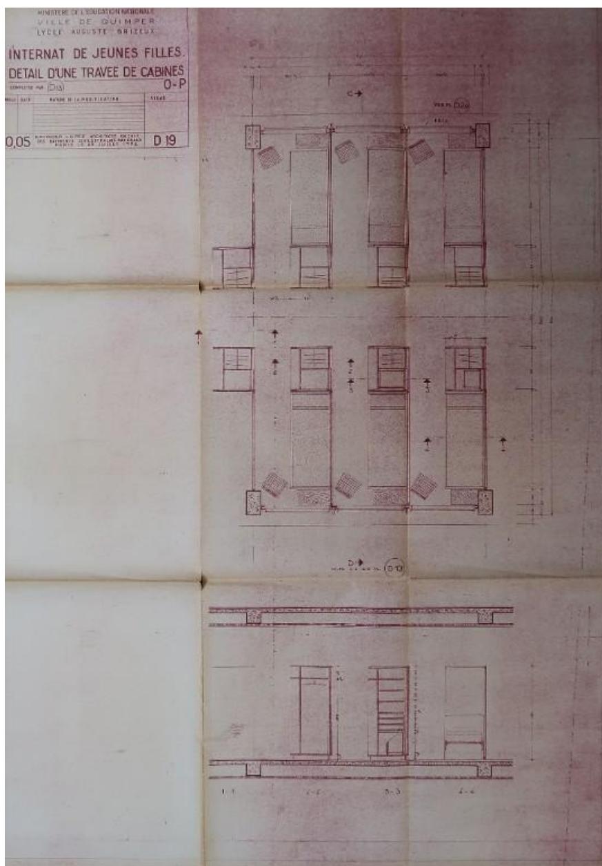
Internat de jeunes filles. Détail d'une travée de cabines. Raymond Lopez, architecte, 1952.
