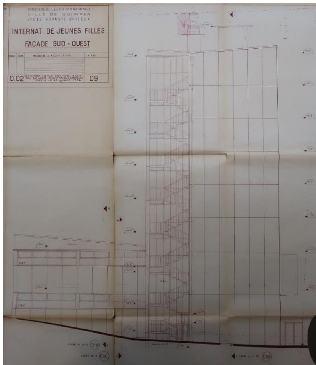
Internat de jeunes filles. Façade sud-ouest. Raymond Lopez, architecte, 1952.
