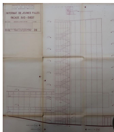
Internat de jeunes filles. Façade sud-ouest. Raymond Lopez, architecte, 1952. Autr. Raymond Lopez IVR53_20252910012A0
