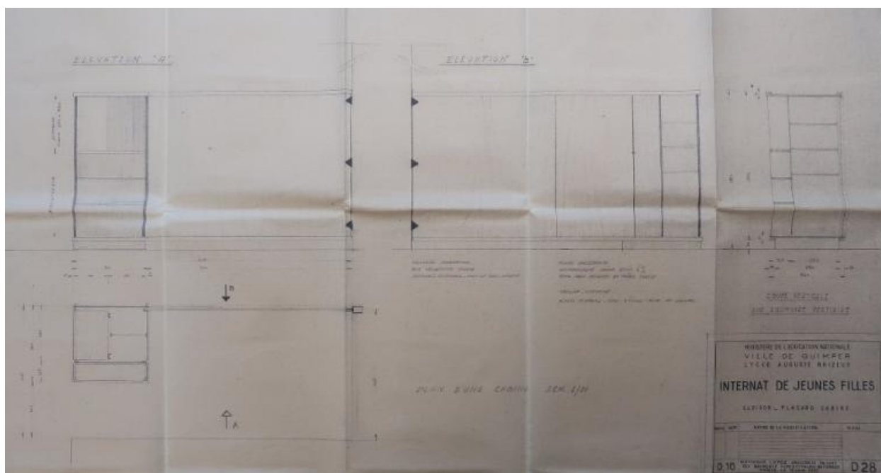
Internat de jeunes filles. Plan d'une 'cabine' ; élévation d'une 'bibliothèque et coiffeuse' ; coupe d'une 'armoire vestiaire'. Raymond Lopez, architecte, 1957.
