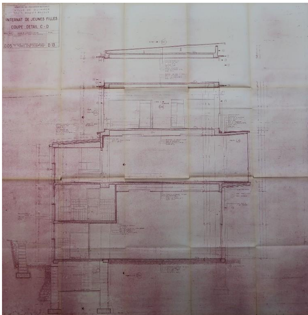
Internat de jeunes filles. Coupe détail. Raymond Lopez, architecte, 1952.
