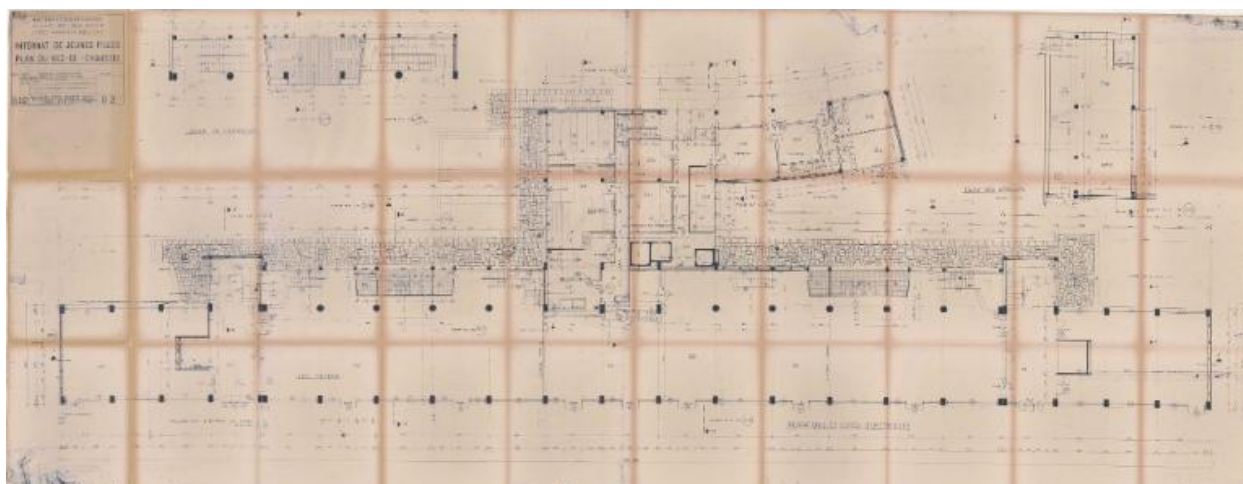
Internat de jeunes filles. Plan du rez-de-chaussée. Raymond Lopez, architecte, 1952.
