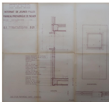
Internat de jeunes filles. Panneau préfabriqué de façade. Raymond Lopez, architecte, 1952. Autr. Raymond Lopez IVR53_20252910020A0
