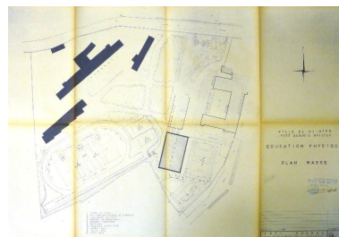
Plan masse de l'établissement, établi par l'architecte Joël Guénec, lors de la construction du gymnase (1962), sur la base du plan de Raymond Lopez. Les bâtiments de l'internat de 1958 figurent en noir. Autr. Joël Guénec IVR53_20172905659NUCA
