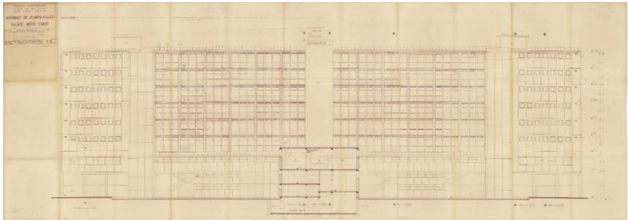
Internat de jeunes filles. Façade nord-ouest. Raymond Lopez, architecte, 1952.
