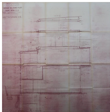
Internat de jeunes filles. Coupe détail. Raymond Lopez, architecte, 1952. Autr. Raymond Lopez IVR53_20252910016A0
