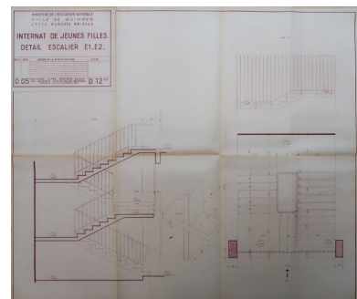
Internat de jeunes filles. Détail escalier E1 - E2. Raymond Lopez, architecte, 1952. Autr. Raymond Lopez IVR53_20252910015A0
