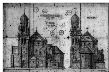
Plan des façades sud et est Repro. Guy Artur IVR53_19813500314P
