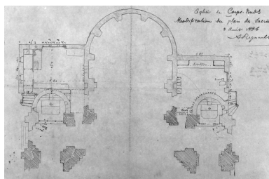
Modification du plan de sacristie. Phot. Guy Artur, Autr. Arthur Regnault IVR53_19953500119V
