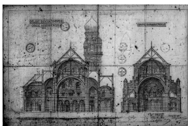
Coupes longitudinale et transversale Repro. Guy Artur IVR53_19813500312P
