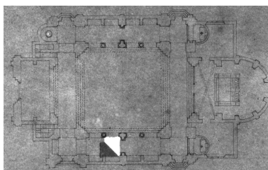
Plan au sol de l'église. Phot. Guy Artur, Autr. Arthur Regnault IVR53_19953500118V
