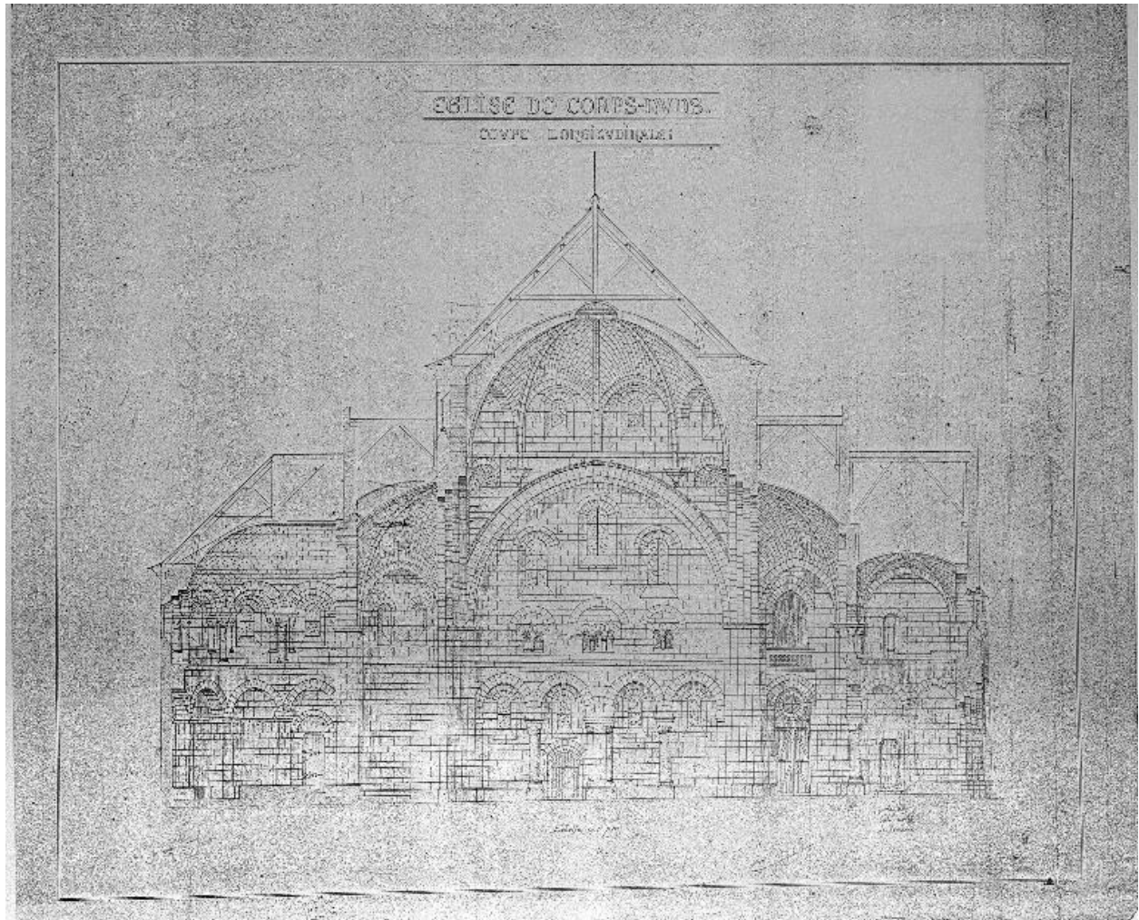
Plan de l'église : coupe longitudinale
