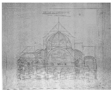
Plan de l'église : coupe longitudinale Repro. Norbert Lambart IVR53_19973500153X
