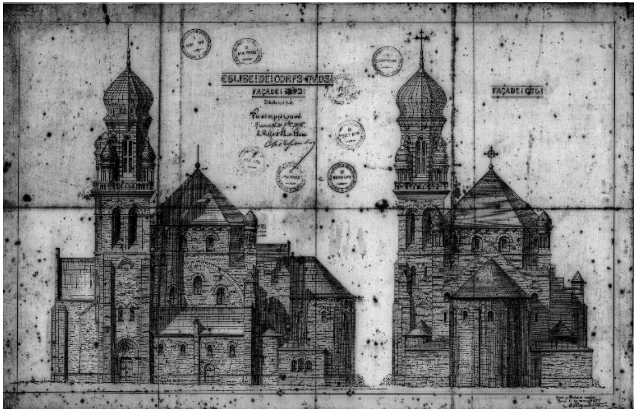
Plan des façades sud et est
